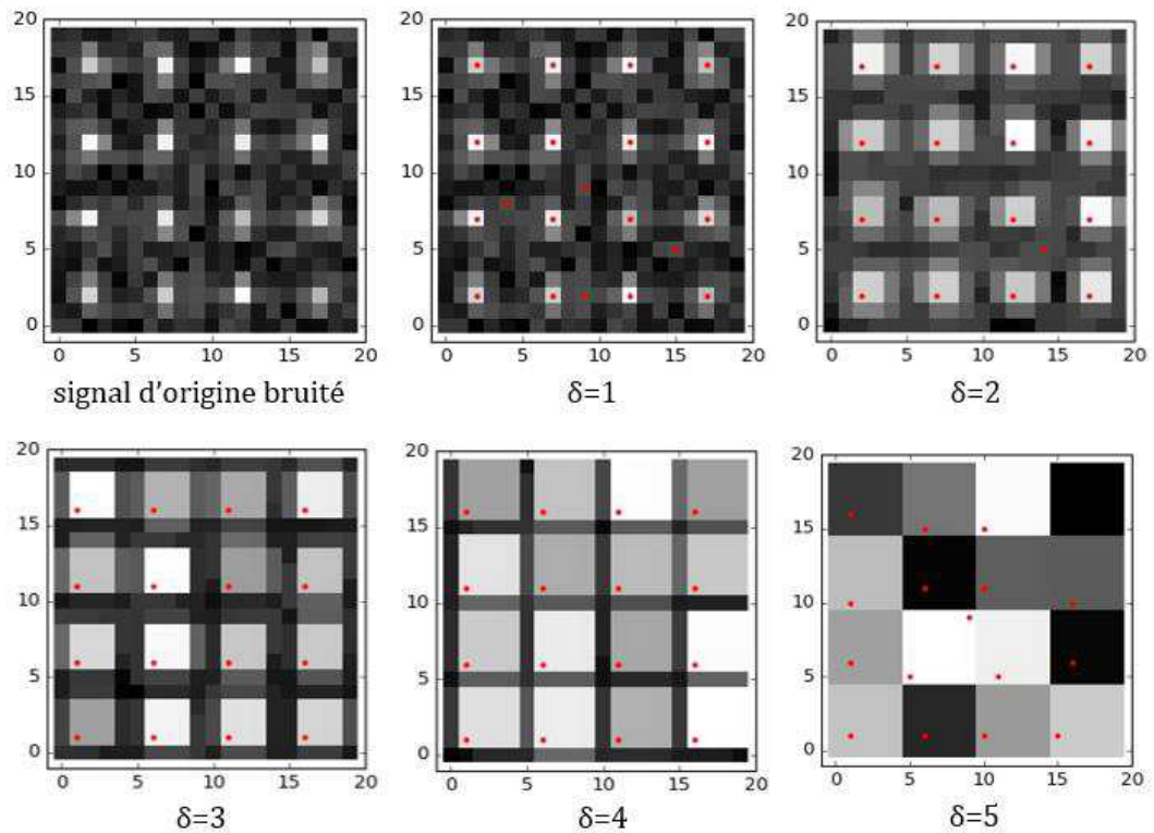
Figure 122. Mise en  vidence de l'influence de la taille d'entr e \delta du filtre de maximum pour la d tection de maximum locaux. Le filtre est appliqu  sur une zone de test compos e de 16 maxima locaux sur une image bruit e. Les points rouges repr sentent les maxima locaux d tect s.
