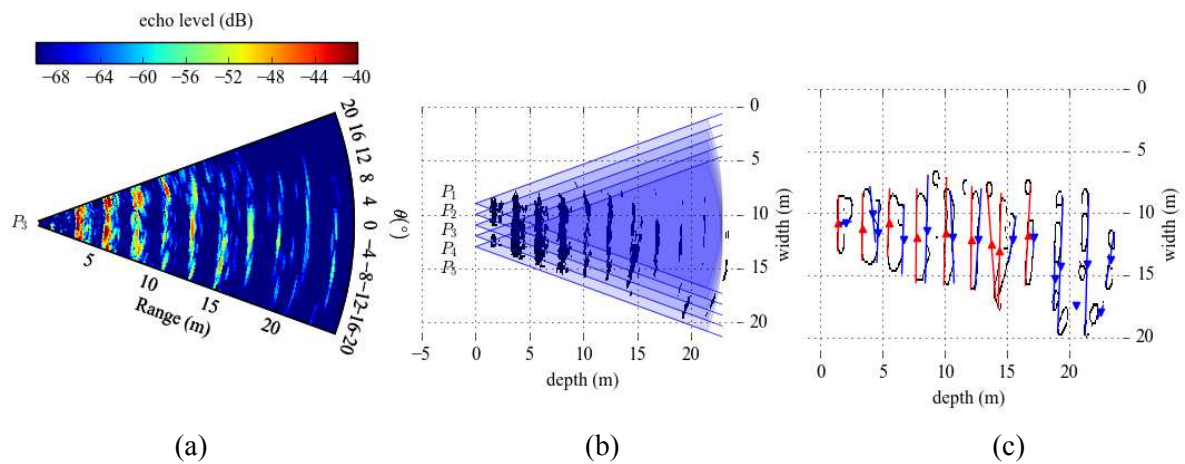
Figure 136. (a) Image radar 2D dans un plan de coupe (R,\theta) en élévation \varphi=7^\circ obtenue à 24GHz en couplage de couplage VV devant le pied de vigne GR n°3 représenté par le point P3 (b) Les niveaux d'échos supérieurs à -60dB (pixels noirs) sont superposés après cinq balayages aux positions P1,P2,P3,P4 et P5. (c) Les orientations des rangées de vignes calculées par une transformée de Hough sont représentées par les lignes rouges (début de rangée) et les lignes bleus (fin de rangée). Les lignes noires représentent les contours de l'image radar après seuillage détectés par un filtre de Canny.
