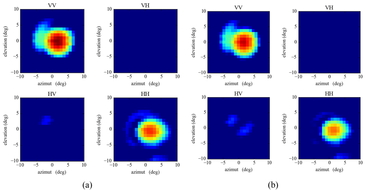
Figure 104. Images radar 2D dans le plan (\theta, \varphi) pour R=1,50\text{m} (soit 20 fois la résolution en profondeur d ) de la sphère métallique de 6,4 cm de diamètre pour : (a) une feuille de plastique sans gouttelettes d'eau (b) une feuille de plastique avec gouttelettes d'eau Echelle : -50dB (bleu) à -30dB (rouge)
