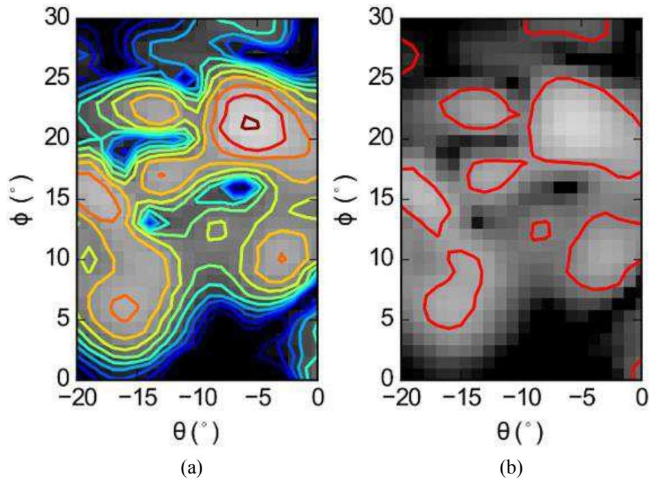
Figure 121. (a) Contours g n r s pour diff rents niveaux d' chos initiaux de -60dB (bleu)   -30dB (rouge) et (b) contours g n r s en appliquant l'algorithme s lectif bas  sur le calcul des maximum locaux. Image radar 2D dans le plan (\theta, \phi) , en R=1,725m (soit 23 fois la r solution en profondeur d ) g n r e avec le radar 24GHz en couplage de polarisation VV.
