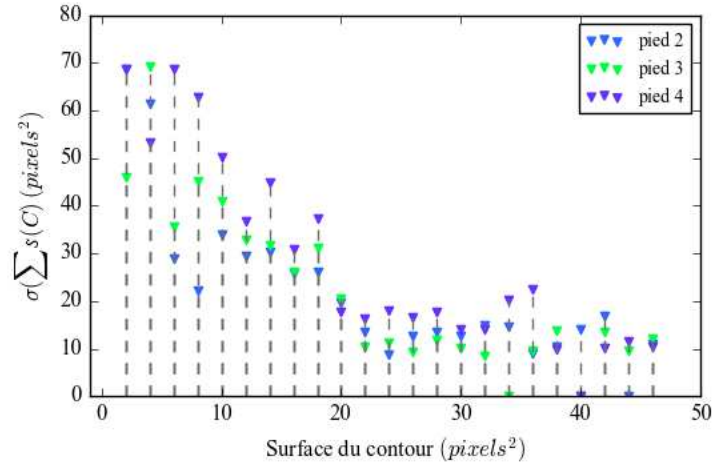
Figure 117. Ecart-type de la somme des surfaces des contours \sigma(\sum_{k=1}^{N_C} s(C_k)) en fonction de la surface des contours pour les trois pieds de variété Merlot.
