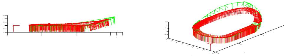
FIGURE 3.9 – La trajectoire estimée par ORBSLAM (vert) sur les images GS générées par Blender. La trajectoire vérité terrain est affichée en rouge. En vue de côté (gauche) une légère dérive de la pose s'observe sur la fin de la trajectoire. En vue du dessus (droite), une dérive de la trajectoire s'observe principalement sur l'axe x et y .
