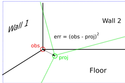
FIGURE 5.5 – Illustration de l'erreur de reprojection entre le point 2D du modèle reprojété (vert) et l'observation (rouge). L'erreur de reprojection correspond à la distance euclidienne au carré.
