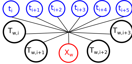
FIGURE 4.9 – Exemple de graphe traduisant l’observation d’un amer X_w dans une image où la pose est contrainte par 4 PC T_{w,i..i+3} et 6 horodatages de PC t_{i..i+6} .
