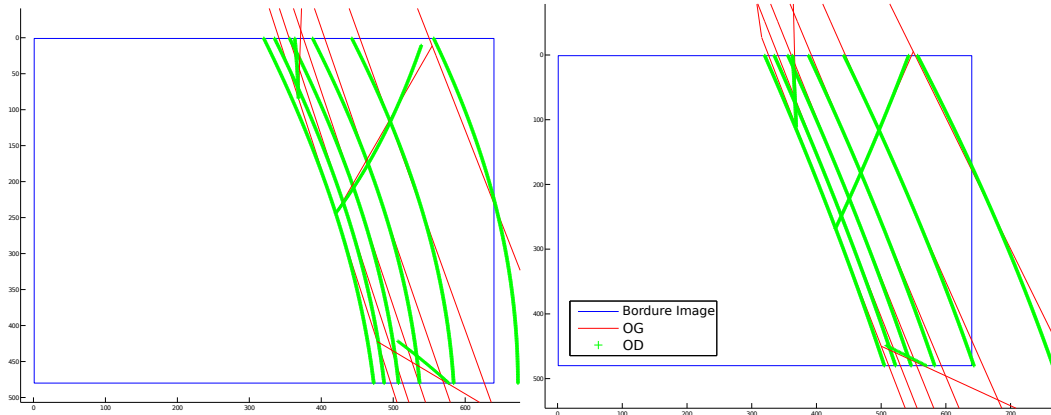
FIGURE 4.19 – Projection d'une grille observée par une caméra en mouvement à l'aide d'un modèle de projection OD(vert) et OG(rouge). A gauche la durée d'exposition de l'image est de 32ms à gauche et 10ms à droite. Ces temps d'exposition correspondent à des temps d'exposition communs respectivement en intérieur et en extérieur.
