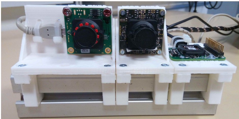
FIGURE 3.11 – Le dispositif permettant d'acquérir des séquences de scènes d'intérieurs. Les deux caméras (OD à gauche et OG à droite) ont des points de vue suffisamment proches pour que leurs images soient comparables. La centrale inertielle à gauche, qui peut être utilisée pour la synchronisation.
