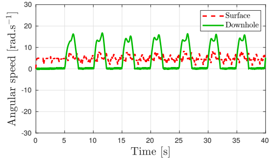
(d) Nonlinear system with \Omega_0 = 5
