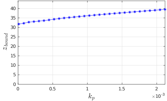
(d) k_i^\phi = 10 , \Omega_0 = 5 and N \in 5 .
