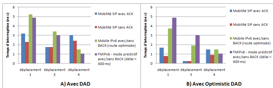
Figure 20. Temps d'interruption ressenti par le MN en tant que récepteur
