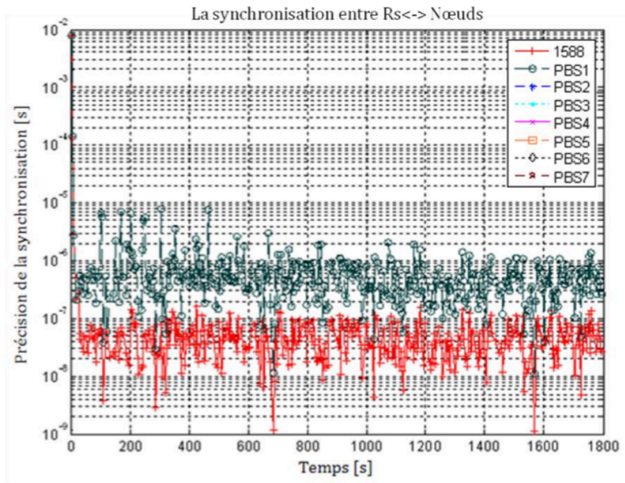
Figure 38 - Synchronisation mesurée pour le protocole IEEE15888-PBS Hybride
