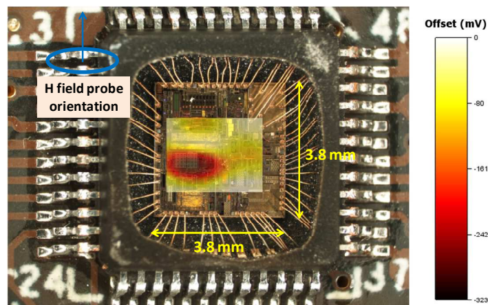
Figure 23 – Cartographie de l'offset induit en sortie du régulateur en fonction de la position de la sonde d'injection ( F_{RF} = 690 \text{ MHz} , P_{RF} = 20 \text{ W} ) [BOY15]
