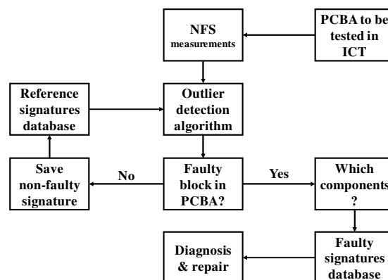
Figure 33 – Méthode de détection proposée de composants défectueux sur circuit imprimé [BEL18]
