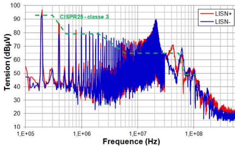
Figure 2 - Exemple de résultat de mesure d'émission conduite d'un équipement électronique
