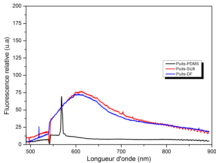
FIGURE 3.52 – Spectre d'auto fluorescence des différents matériaux à travers les puits des puces PDMS/Verre, SU8/Verre et DF/Verre. L'excitation a été faite à 545nm et la détection a été enregistrée entre 500 et 900nm
