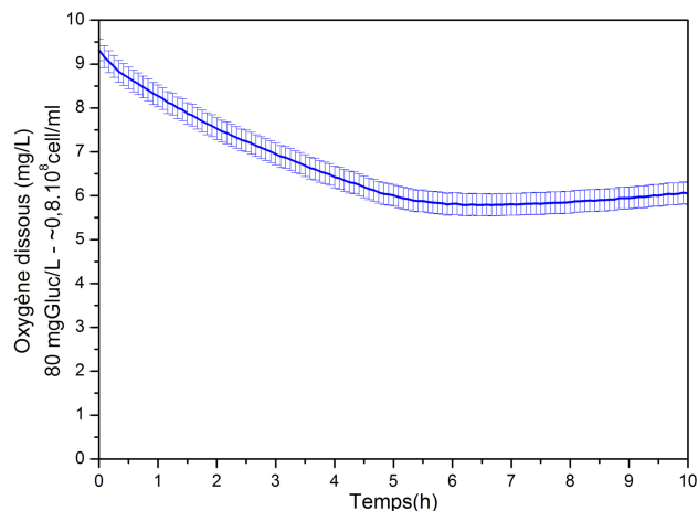
FIGURE 2.4 – Reproductibilité des mesures en milieu M9, pour une concentration de 80 mg-Gluc/L et une population bactérienne ( E.coli ) de 0,8.10 8 cell/mL
