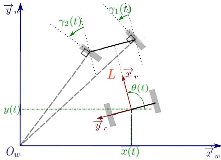
(a) Modèle de véhicule à direction de type Ackermann
