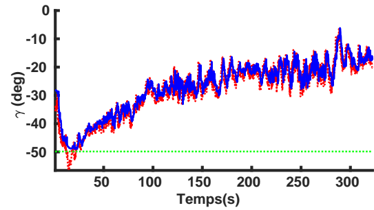
(d) Ligne bleue continue : \gamma(t) - Ligne rouge pointillée : \gamma^*(t) - Ligne verte pointillée : \gamma_{MIN}
