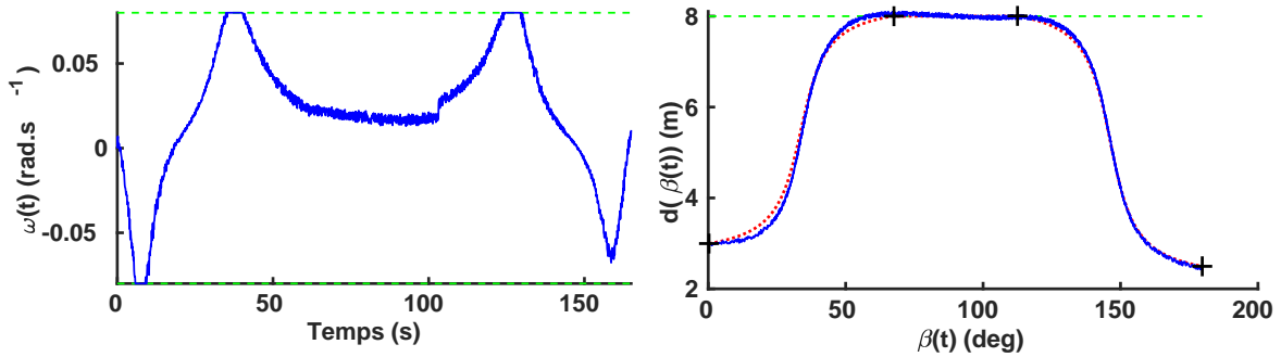
(a) Vitesse angulaire du robot - Ligne bleue continue : \omega(t) (b) Profil en distance - Ligne bleue continue : d(t) - Ligne rouge pointillée : d(\beta(t))
