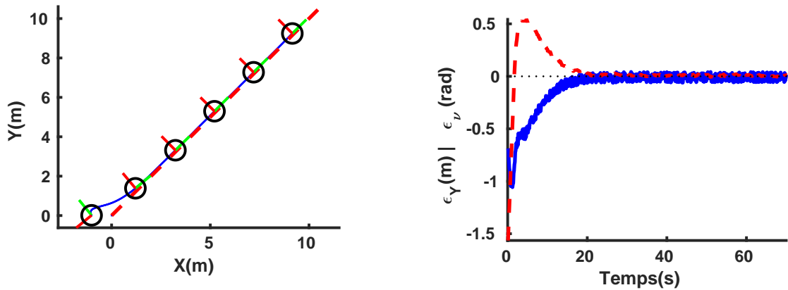
(a) Trajectoire du robot - Ligne continue bleue : Position du robot - Ligne tiretée rouge : Ligne de référence
