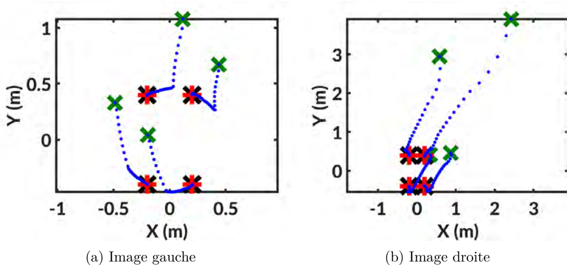
FIGURE 3.8 – Évolution des indices visuels dans les images - Croix vertes : Position initiale - Croix noires : Position désirée ( S^* ) - Croix rouges : Position finale - Points bleus : Trajectoire des indices visuels
