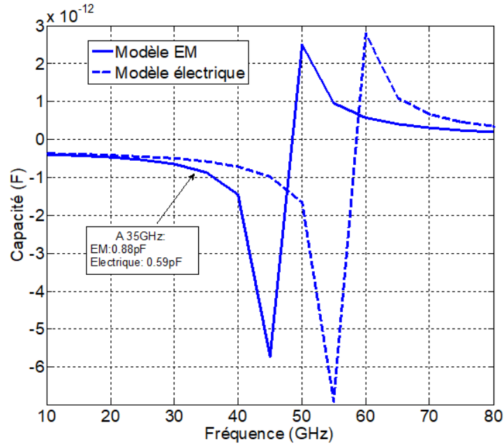
FIGURE 2.4 – Comportements fréquentiels des modèles électrique et EM d'une capacité MIM de valeur nominale 0.38pF
