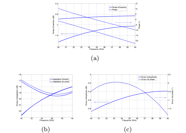
FIGURE 2.10 – Cellule 11.25° single-ended (a) pertes d'insertion et phase (b) niveaux d'adaptation et (c) erreurs fonctionnelles
