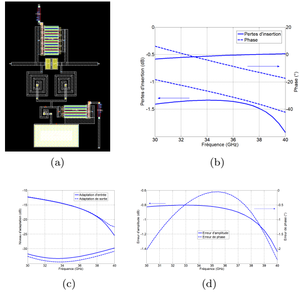
FIGURE 2.11 – Cellule 22.5^\circ single-ended (a) dessin des masques de la cellule et performances en (b) pertes d'insertion et phase (c) niveaux d'adaptation et (d) erreurs fonctionnelles
