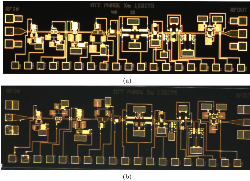
FIGURE 4.4 – Core-chips single-ended fabriqués (a) première version 3.13 \times 1.1 \text{mm}^2 (b) version avec la polarisation corrigée 3.2 \times 1.1 \text{mm}^2
