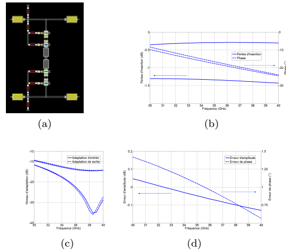
FIGURE 2.30 – Cellule 1dB différentielle (a) dessin des masques de la cellule et performances en (b) pertes d’insertion et phase (c) niveaux d’adaptation et (d) erreurs fonctionnelles
