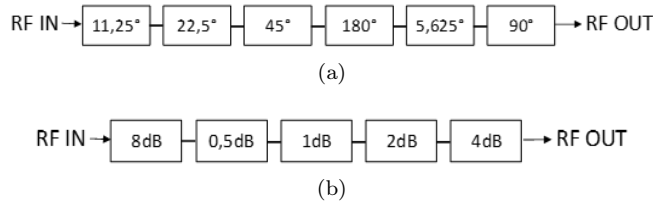
FIGURE 3.21 – Agencement de cellules (a) de déphasage (b) d'atténuation présentant l'erreur de phase moyenne la plus faible
