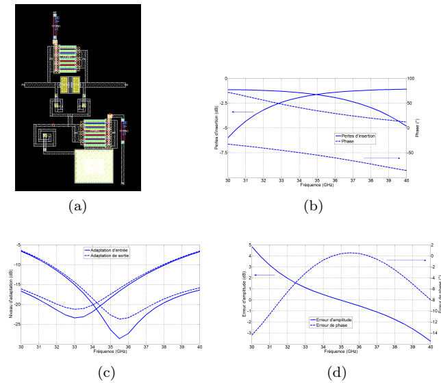
FIGURE 2.13 – Cellule 90^\circ single-ended (a) dessin des masques de la cellule et performances en (b) pertes d'insertion et phase (c) niveaux d'adaptation et (d) erreurs fonctionnelles
