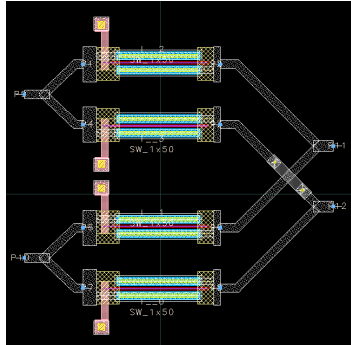
FIGURE 2.22 – Dessin des masques utilisés lors de la simulation EM de la cellule 180°
