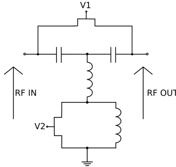
FIGURE 1.11 – Topologie en T passe-haut avec circuit bouchon
