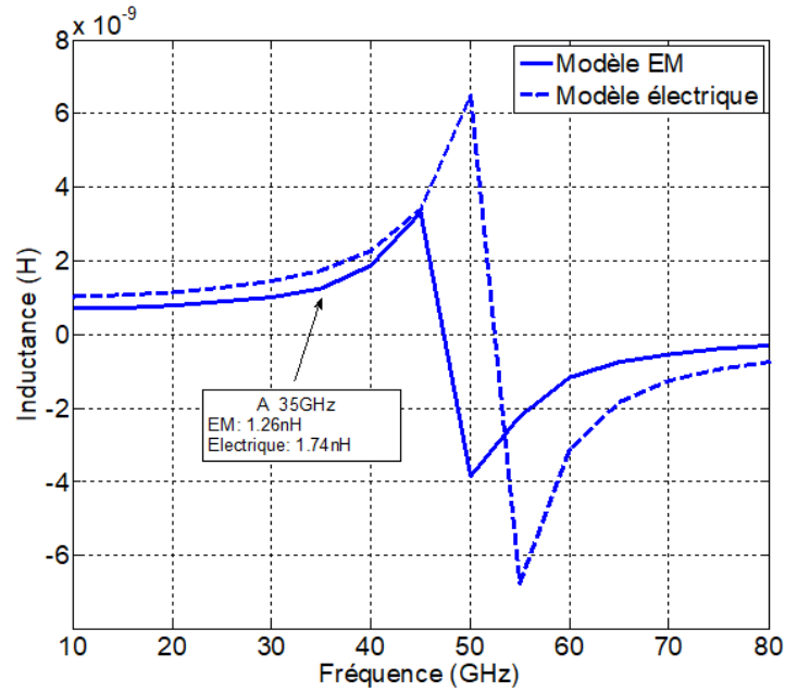
FIGURE 2.5 – Comportements fréquentiels des modèles électrique et EM d'une inductance de valeur nominale 0.99nH
