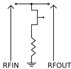
FIGURE 1.16 – Mise en série d'une résistance pour atténuer le signal incident
