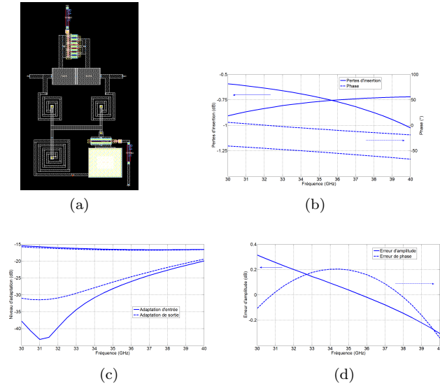
FIGURE 2.12 – Cellule 45^\circ single-ended (a) dessin des masques de la cellule et performances en (b) pertes d'insertion et phase (c) niveaux d'adaptation et (d) erreurs fonctionnelles
