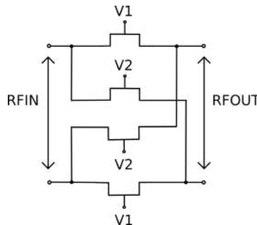
FIGURE 2.20 – Schéma électrique de la cellule 180° différentielle
