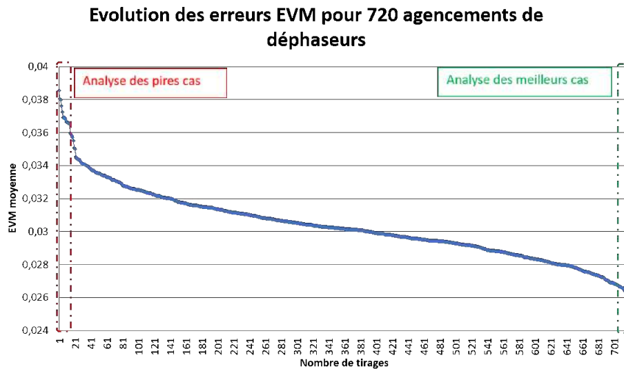
FIGURE 3.16 – Evolution de l'EVM moyen pour 720 agencements de 6 cellules de déphasage
