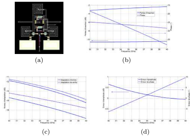
FIGURE 2.19 – Cellule 8dB single-ended (a) dessin des masques de la cellule et performances en (b) pertes d'insertion et phase (c) niveaux d'adaptation et (d) erreurs fonctionnelles
