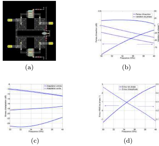
FIGURE 2.25 – Cellule 22.5^\circ différentielle (a) dessin des masques de la cellule et performances en (b) pertes d'insertion et phase (c) niveaux d'adaptation et (d) erreurs fonctionnelles
