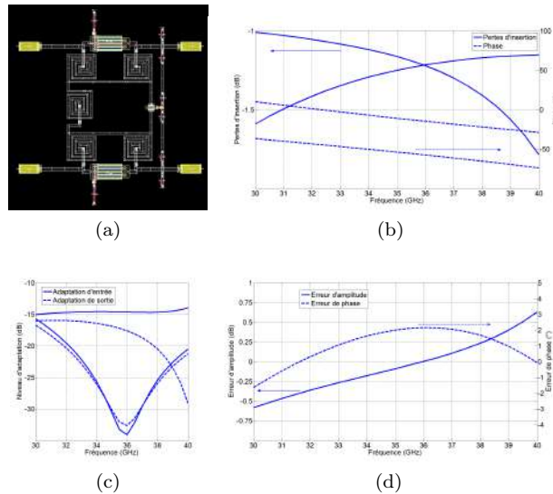
FIGURE 2.26 – Cellule 45^\circ différentielle (a) dessin des masques de la cellule et performances en (b) pertes d'insertion et phase (c) niveaux d'adaptation et (d) erreurs fonctionnelles
