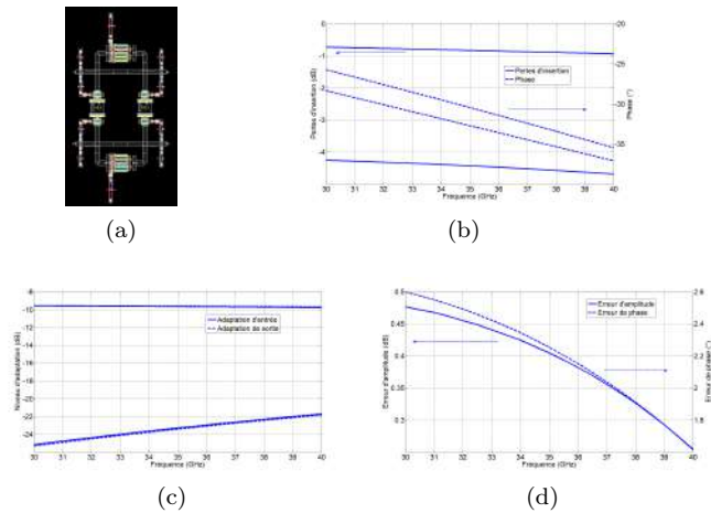
FIGURE 2.32 – Cellule 4dB différentielle (a) dessin des masques de la cellule et performances en (b) pertes d’insertion et phase (c) niveaux d’adaptation et (d) erreurs fonctionnelles
