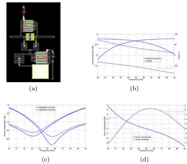
FIGURE 2.13 – Cellule 90° single-ended (a) dessin des masques de la cellule et performances en (b) pertes d'insertion et phase (c) niveaux d'adaptation et (d) erreurs fonctionnelles
