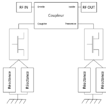
FIGURE 1.15 – Topologie de déphaseur dit "réflectif"
