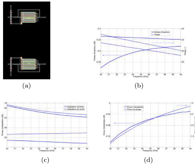
FIGURE 2.23 – Cellule 5.625^\circ différentielle (a) dessin des masques de la cellule et performances en (b) pertes d'insertion et phase (c) niveaux d'adaptation et (d) erreurs fonctionnelles
