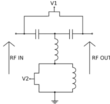
FIGURE 1.11 – Topologie en T passe-haut avec circuit bouchon
