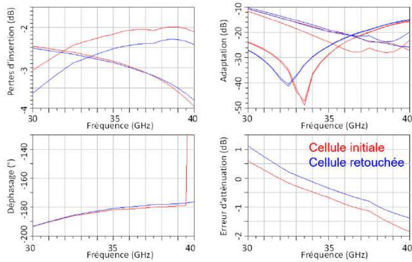
FIGURE 3.6 – Retouche de la cellule 180^\circ single ended avec en rouge les performances initiales et en bleu les performances finales
