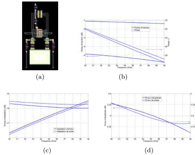
FIGURE 2.18 – Cellule 4dB single-ended (a) dessin des masques de la cellule et performances en (b) pertes d'insertion et phase (c) niveaux d'adaptation et (d) erreurs fonctionnelles
