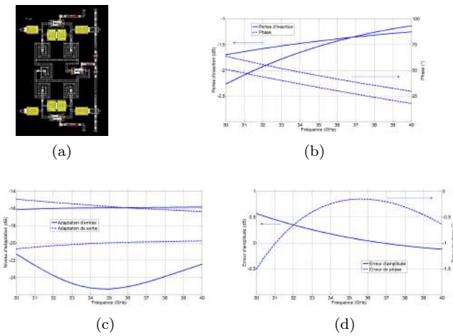
FIGURE 2.24 – Cellule 11.25^\circ différentielle (a) dessin des masques de la cellule et performances en (b) pertes d'insertion et phase (c) niveaux d'adaptation et (d) erreurs fonctionnelles
