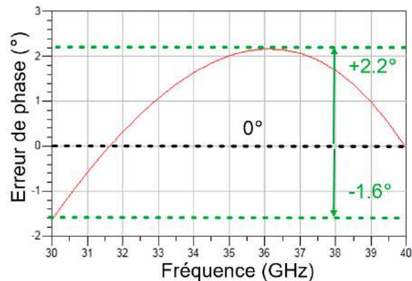
FIGURE 1.21 – Exemple de profil d'erreur pour une cellule de déphasage, en noir le profil d'erreur plat, en vert les erreurs maximales et en rouge l'erreur de phase
