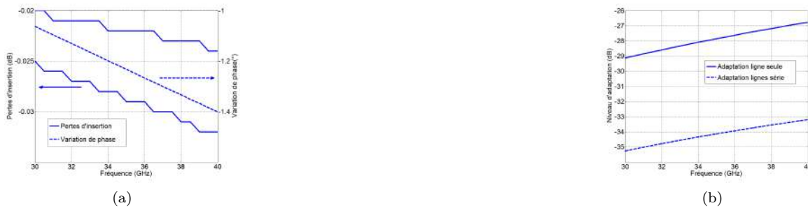
FIGURE 3.3 – Simulation pour apprécier l'effet des ports de connexion sur les résultats de simulation
