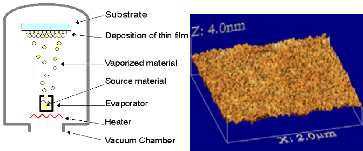
Figure 1.3. Schéma de principe de la sublimation sous ultravide et topographie AFM d'une couche mince du complexe \text{Fe}(\text{phen})_2(\text{NCS})_2 obtenu par évaporation.
