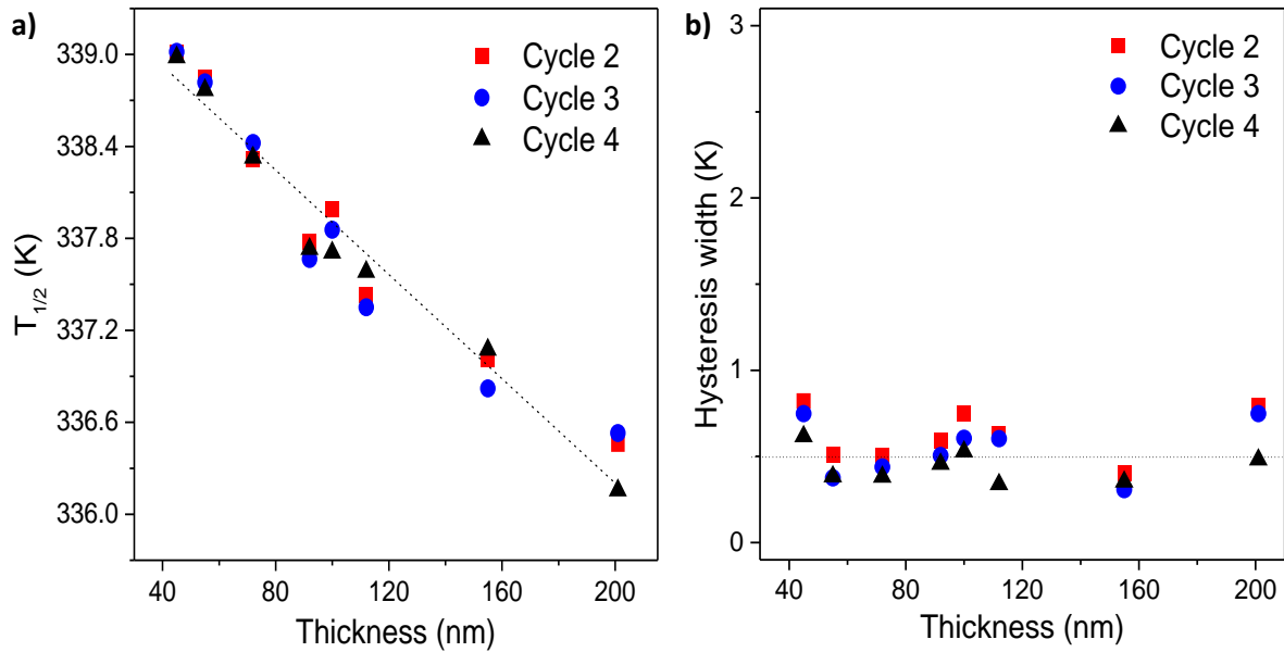
Figure 3.3: Evolution (a) de la température de transition et (b) de la largeur du cycle d'hystérésis thermique en fonction de l'épaisseur du film de [Fe(HB(tz) 3 ) 2 ] pour les différents cycles de chauffage / refroidissement. (Les lignes en pointillés servent de guide pour les yeux.)
