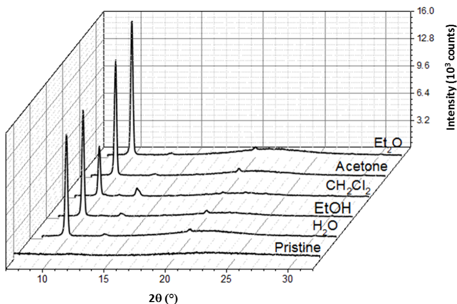
Figure 2.4: Diffractogrammes RX de films du composé [\text{Fe}(\text{HB}(\text{tz})_3)_2] exposés à différents solvants.
