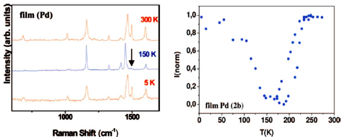
Figure 1.4: Spectres Raman d'une couche mince du composé \{\text{Fe}(\text{azpy})[\text{Pd}(\text{CN})_4]\} enregistrés à différentes températures et la courbe de transition de spin extraite de ces spectres.
