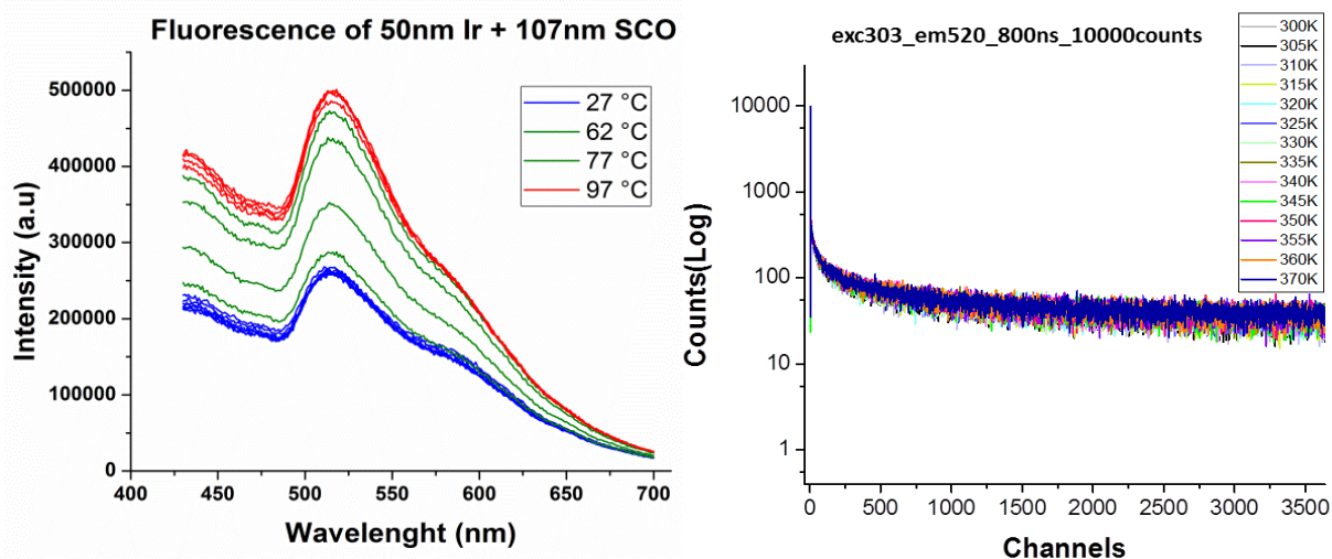
Figure 4.2: Caractérisation du film bicouche d'Ir(PPy) 3 et de [Fe(HB(tz) 3 ) 2 ]. (Figure à gauche) Spectres d'émission, en fonction de la température, obtenus par excitation du complexe d'iridium à 300 nm. (Figure à droite) courbes de décroissance de la luminescence en fonction de la température enregistrées lors des premiers 800 ns de la décroissance.
