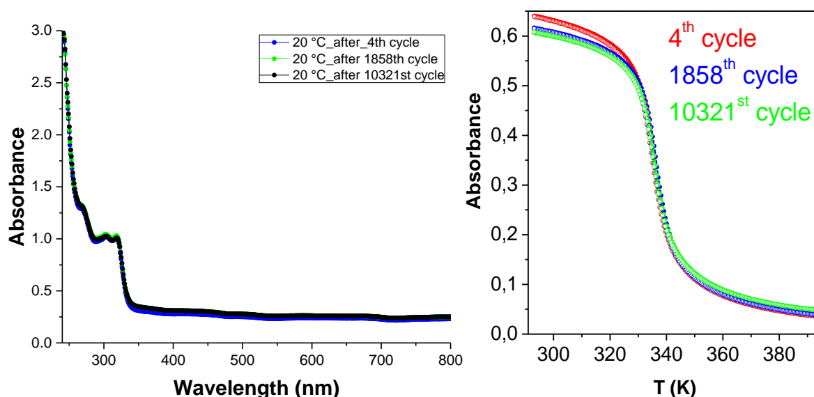
Figure 3.2: (Gauche) Spectres d'absorption et (droite) courbes de transition de spin thermique d'un film de [\text{Fe}(\text{HB}(\text{tz})_3)_2] après différents nombres de cycle thermiques consécutifs.
