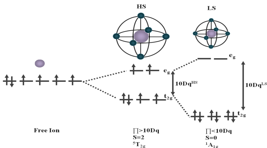
Figure 1.1. Levée de dégénérescence et configuration électronique des états HS et BS dans le cas d'un complexe de Fe^{II} avec un environnement octaédrique.
