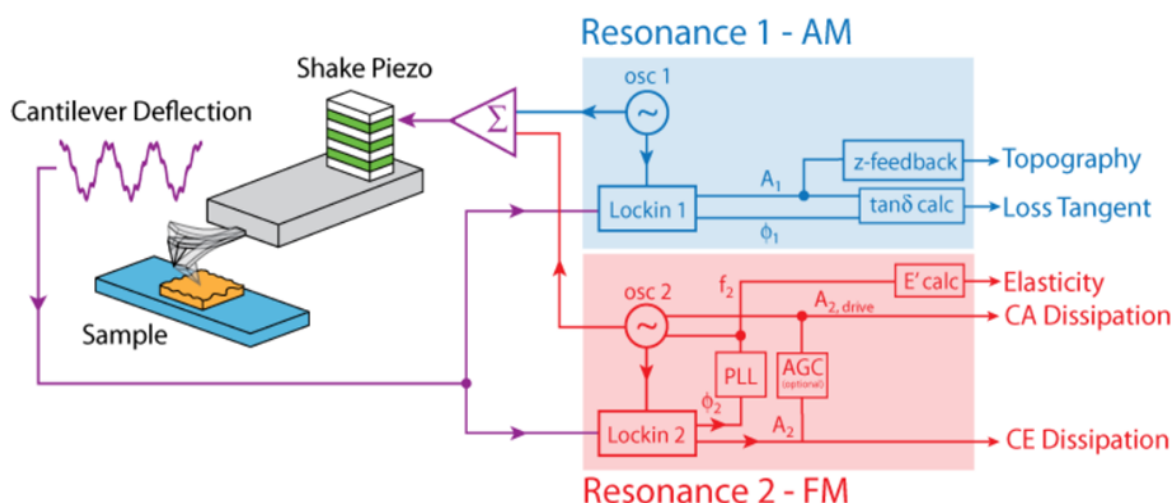
Figure 5.1: Représentation schématique du principe de fonctionnement de l'AFM en mode multi-fréquence (AMFM mode), où deux excitations sinusoïdales sont envoyées vers la pointe AFM (en bleu et en rouge).
