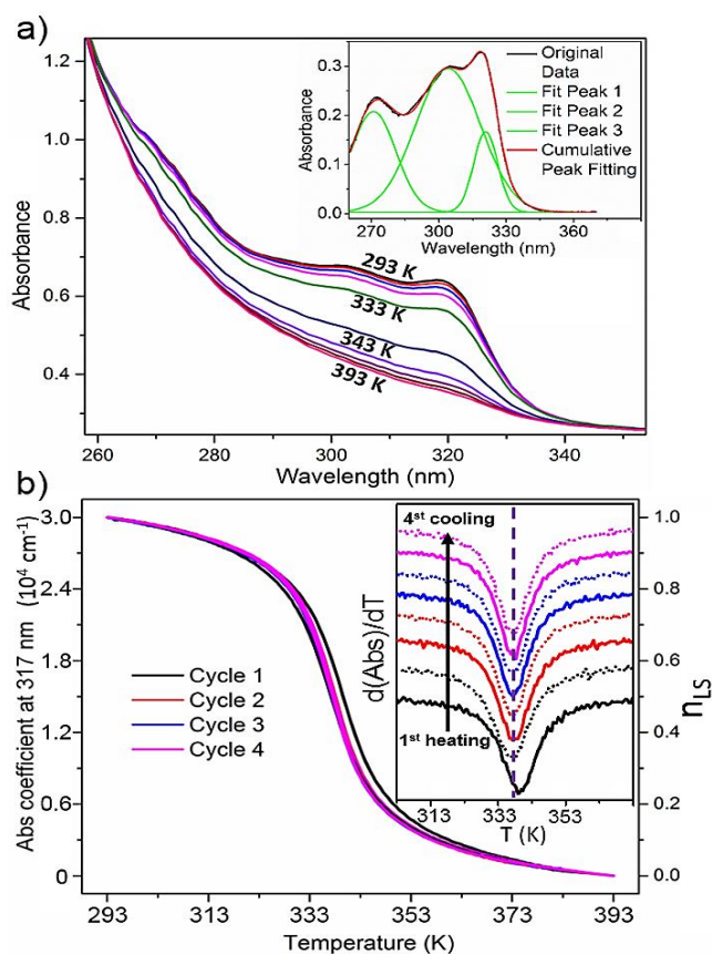
Figure 2.3: (a) Spectre d'absorbance pour un film cristallin de 90 nm d'épaisseur du composé [\text{Fe}(\text{HB}(\text{tz})_3)_2] obtenu à différentes températures lors du chauffage (b) Variation thermique de l'absorbance à 317 nm au cours de 4 cycles thermiques mesurés à 1 K/min.
