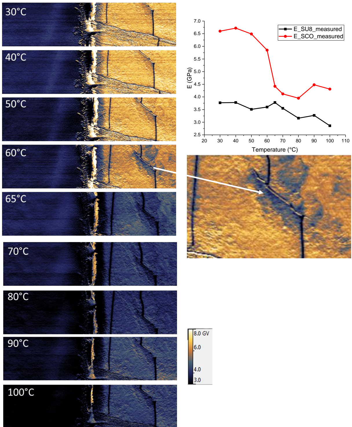
Figure 5.3: Cartographie du module d'Young (en GPa) du matériaux SU-8 and [\text{Fe}(\text{HB}(\text{tz})_3)_2] pour différentes températures sélectionnées. La taille des images est de 14 \mu\text{m} \times 3.5 \mu\text{m} . L'agrandissement de l'image correspondant à la température de 60^{\circ}\text{C} montre la surprenante coexistence des phases bas spin (couleur or) et haut spin (couleur bleue). La dépendance thermique du module d'Young moyen obtenue à partir des images AFM en mode multi-fréquence est également représentée.
