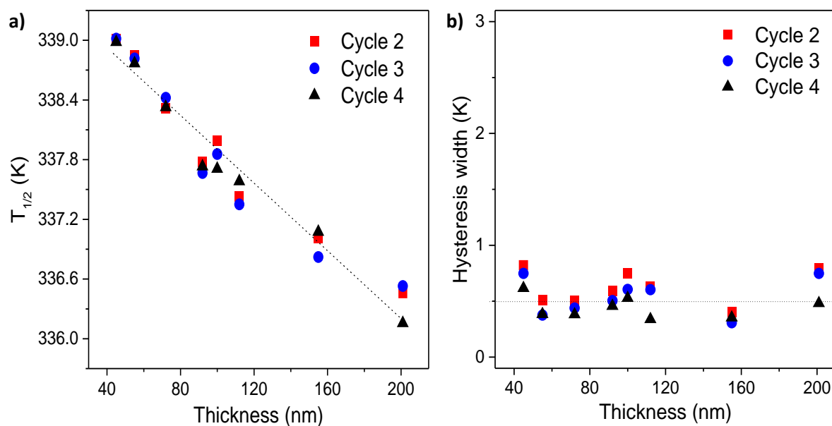
Figure 3.3: Evolution (a) de la température de transition et (b) de la largeur du cycle d'hystérésis thermique en fonction de l'épaisseur du film de [Fe(HB(tz) 3 ) 2 ] pour les différents cycles de chauffage / refroidissement. (Les lignes en pointillés servent de guide pour les yeux.)
