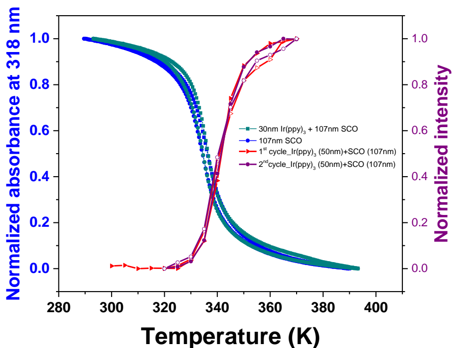
Figure 4.3: Dépendances thermiques normalisées de l'absorbance UV et de l'intensité de l'émission lumineuse du film bicouche (30 + 107 nm d'épaisseur, excitation: 300 nm, émission 520 nm).
