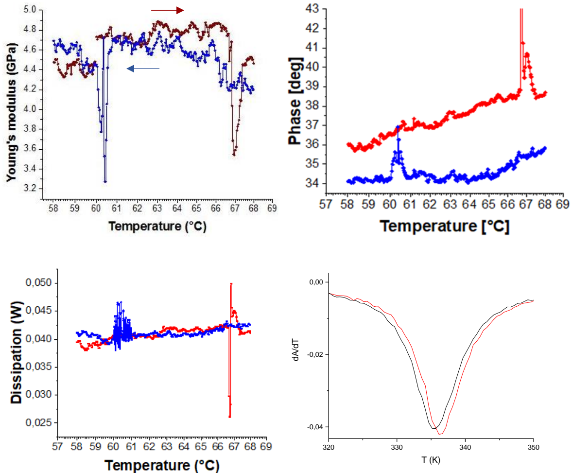
Figure 5.2: Evolution avec la température du (a) Module d'Young, (b) de la phase et (c) de la dissipation pour un film mince de 100nm du composé [\text{Fe}(\text{HB}(\text{tz})_3)_2] obtenue par mesure AFM en mode multi-fréquence. La courbe rouge (resp. bleu) représente la phase de chauffage (resp. la phase de refroidissement). (d) Dérivée de la courbe de transition de spin du même film obtenue par mesures d'absorbance UV.
