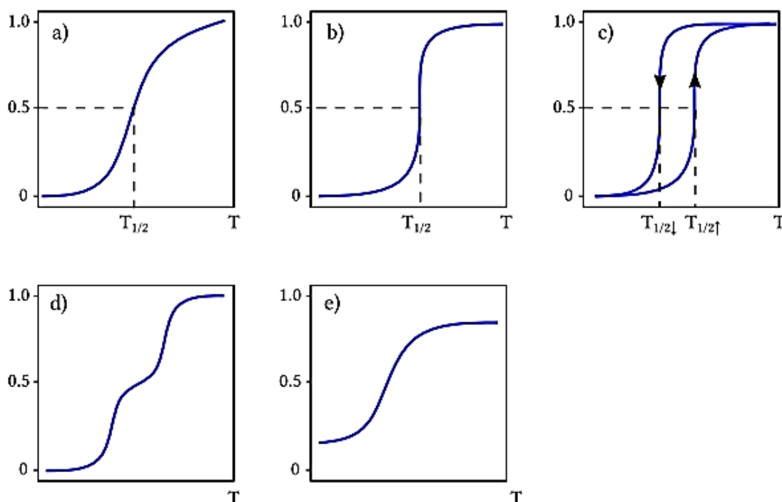
Figure 1.2. Principaux types de transitions de spin thermiques, représentant la fraction HS en fonction de la température : (a) transition de spin graduelle, (b) transition de spin abrupte, (c) transition de spin avec cycle d'hystérésis, (d) transition de spin en deux étapes et (e) transition de spin incomplète.
