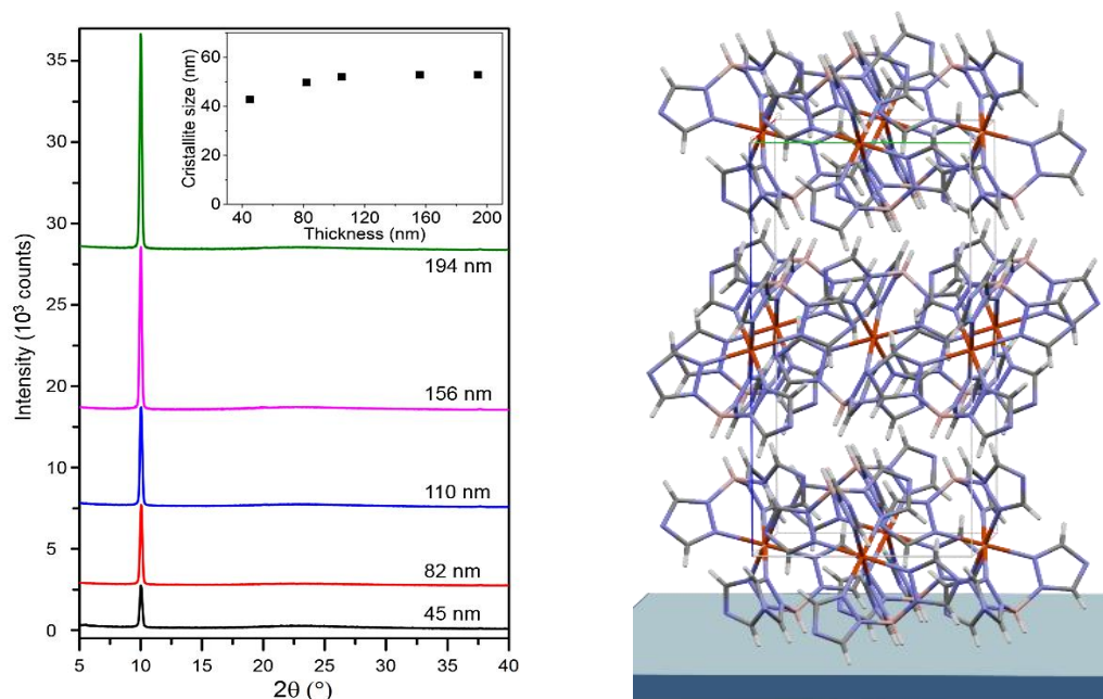
Figure 2.2: Diffractogrammes des rayons X du film cristallin du composé [\text{Fe}(\text{HB}(\text{tz})_3)_2] pour différentes épaisseurs. La structure du film orienté est également montrée.
