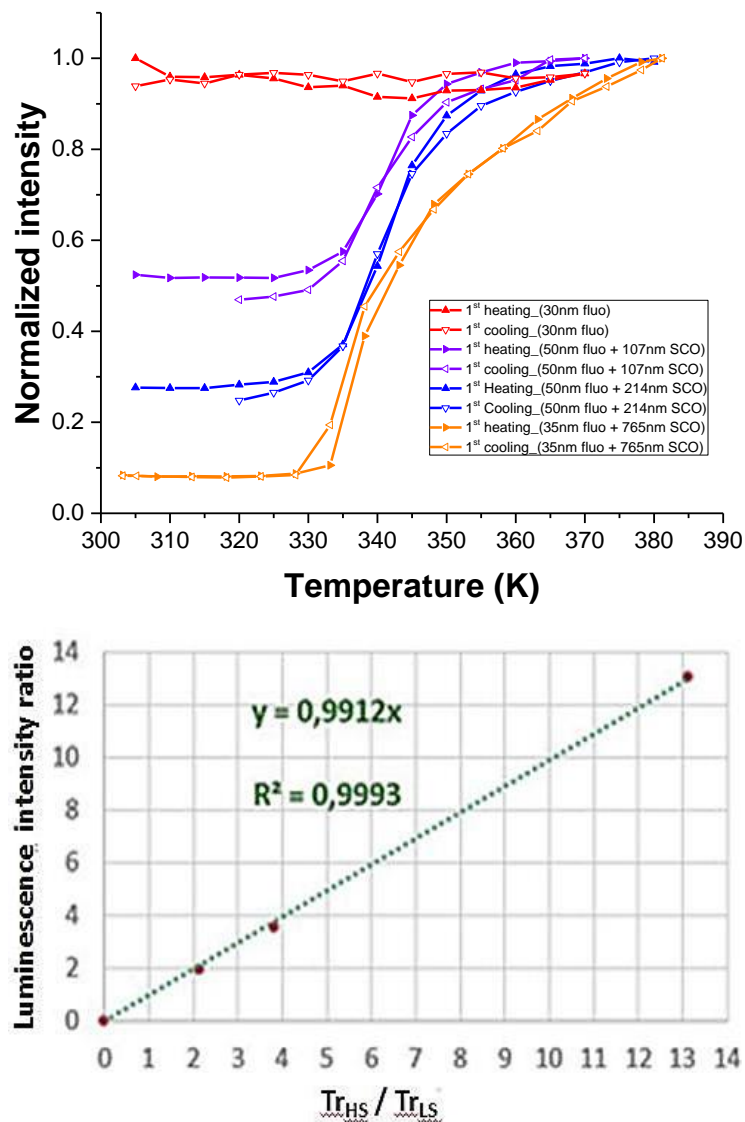
Figure 4.4: (Figure en haut) Dépendance thermique normalisée de l'intensité de la luminescence pour différentes épaisseurs de la couche de complexe à TS dans les films bicouches TS-luminescent. (Figure en bas) tracé du ratio de l'intensité de la luminescence en fonction du ratio de la transmittance du complexe dans les états HS et BS.
