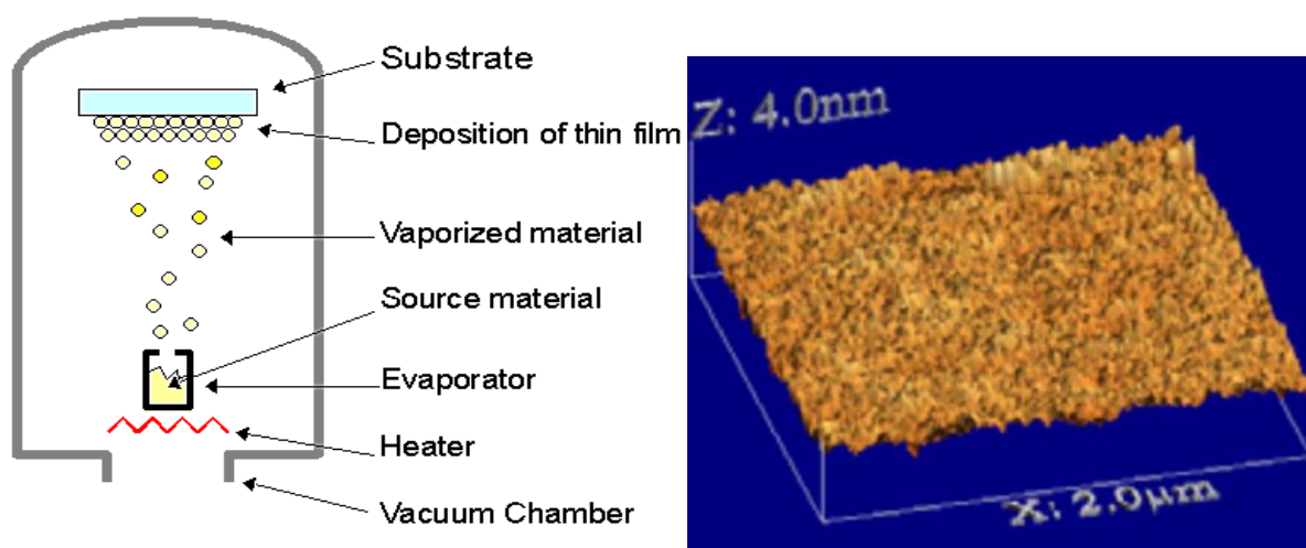
Figure 1.3. Schéma de principe de la sublimation sous ultravide et topographie AFM d'une couche mince du complexe \text{Fe}(\text{phen})_2(\text{NCS})_2 obtenu par évaporation.
