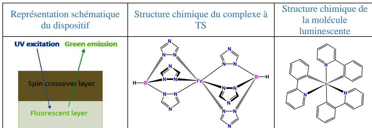
Figure 4.1: Représentation schématique du dispositif et structures chimiques des complexes de fer et d'iridium.
