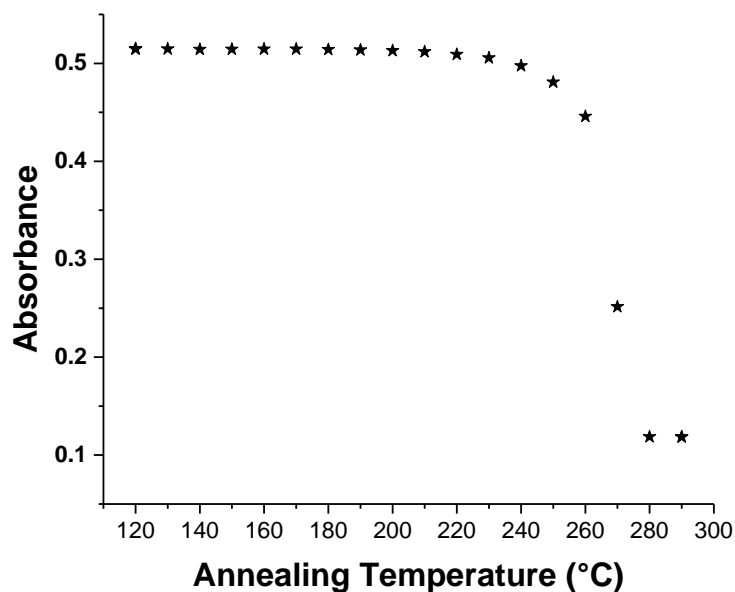
Figure 3.1: Évolution de l'absorbance optique (à 317 nm) à température ambiante d'un film mince de [\text{Fe}(\text{HB}(\text{tz})_3)_2] de 125 nm d'épaisseur en fonction de la température de recuit.
