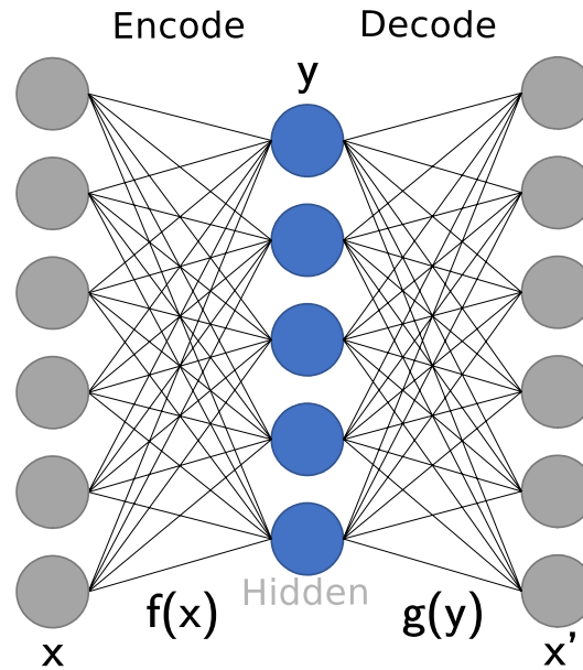
FIGURE 3.4 – Exemple d'auto-encodeur
