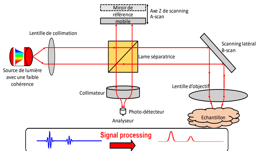
Figure I-2 : Principe de base d'un système de type TD-OCT utilisant une source de faible cohérence
