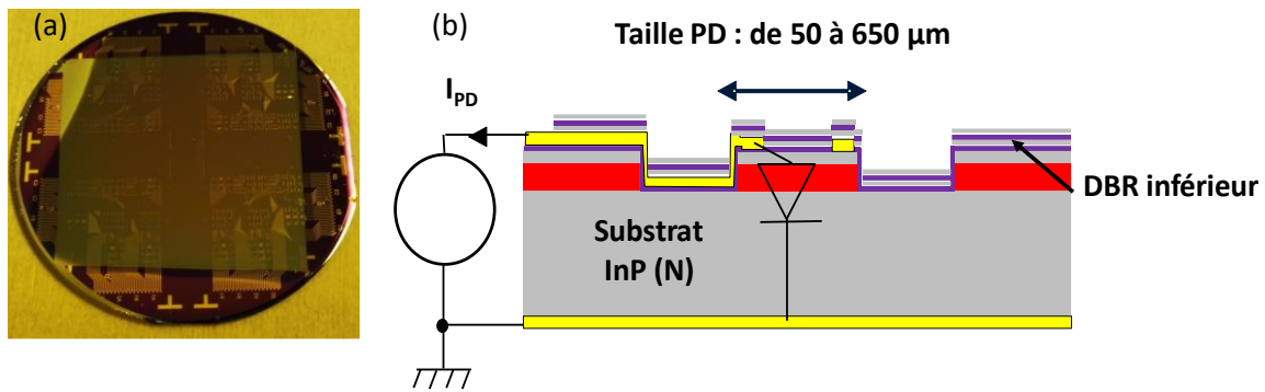
Figure III-6 : (a) Photo d'un wafer 2 pouces après la fabrication des PD et (b) dépôt du DBR et schéma d'une vue en coupe d'une PD après le dépôt du DBR inférieur. (Institut FOTON)
