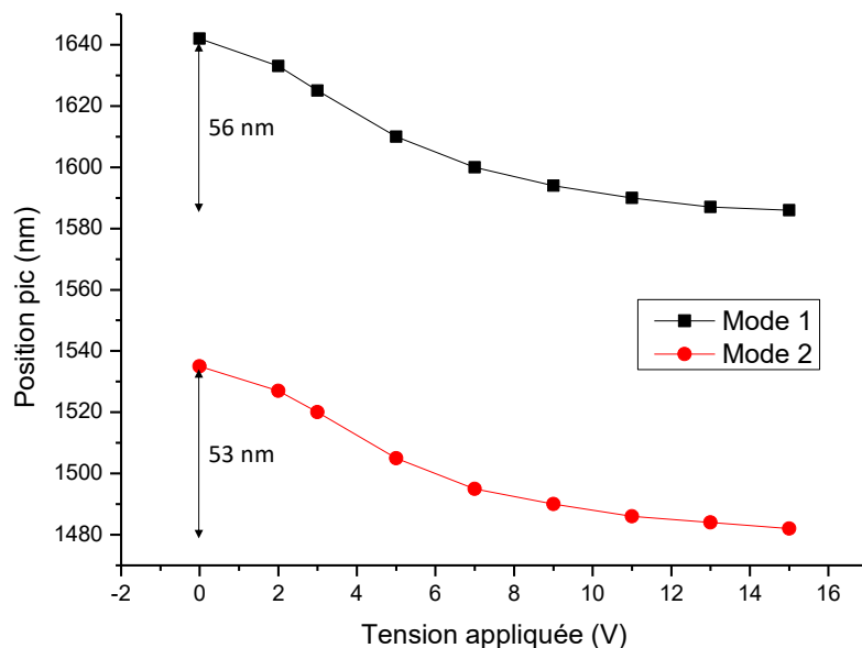
Figure III-13 : Courbe d'accordabilité sur une photodiode après un traitement \text{SiO}_2 de 5 minutes
