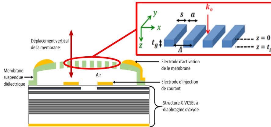
Figure I-21 : Schéma d'une structure VCSEL avec un HCG suspendu sur un MEMS diélectrique. Insert : principe d'un HCG de période A et d'épaisseur t_g : largeur de la bande de matériau de haut indice, a : largeur de la bande de matériau de faible indice (air)
