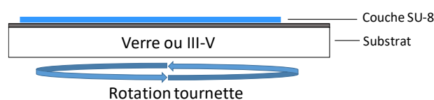
Figure II-27 : Enduction de SU-8 pour la réalisation de l'ancrage ou pour le scellement
