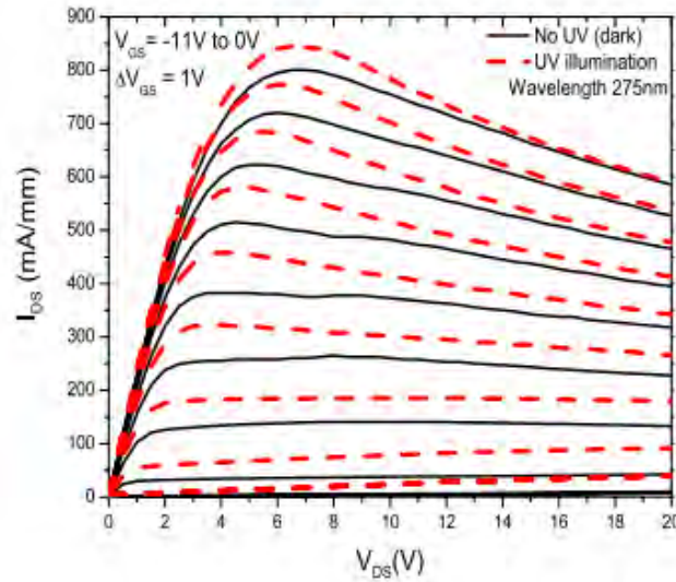
Figure 2.24 Caractéristiques de sortie I-V d'un HEMT AlGaN / GaN, dans l'obscurité et sous un éclairage UV [140].
