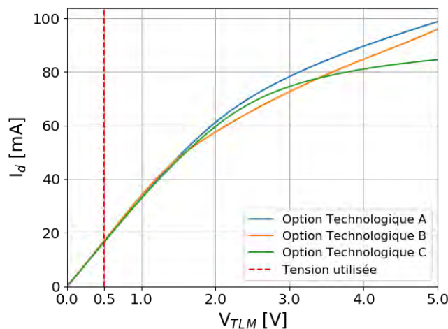
Figure 2.34 Caractéristiques I-V pour trois échantillons de chaque option technologique, à T = 25 °C, L_i = 4 \mu m. La tension sélectionnée est de 500 mV pour toutes les mesures dans cette partie (ligne rouge en pointillé).
