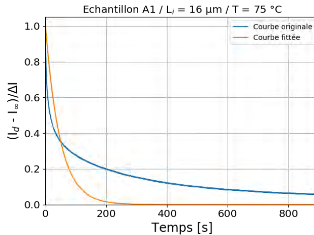
Figure 3.3 Exemple d'un ajustement mono-exponentielle appliqué sur des données expérimentales effectuées sur l'échantillon A1, pour L_i = 16 \mu\text{m} et T = 75 \text{ °C} .
