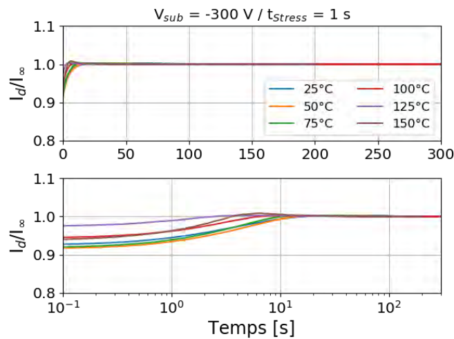
Figure 2.17 Courant de drain normalisé en fonction de temps, mesuré après le stress sous différentes températures, avec V_{TLM} = 200 \text{ mV} ; V_{sub} = -500 \text{ V} ; t_{Stress} = 1 \text{ s} ; sous la présence d'une source lumineuse ; courbes du haut en échelle linéaire, courbes du bas en échelle logarithmique.
