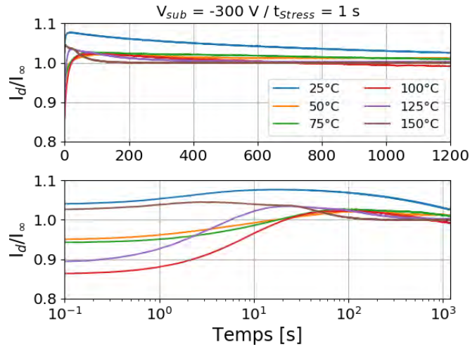
Figure 2.16 Courant de drain normalisé en fonction de temps, mesuré après le stress sous différentes températures, avec V_{TLM} = 200 \text{ mV} ; V_{sub} = -300 \text{ V} ; t_{Stress} = 1 \text{ s} ; dans l'obscurité ; station sous pointes Cascade ; courbes du haut en échelle linéaire, courbes du bas en échelle logarithmique.
