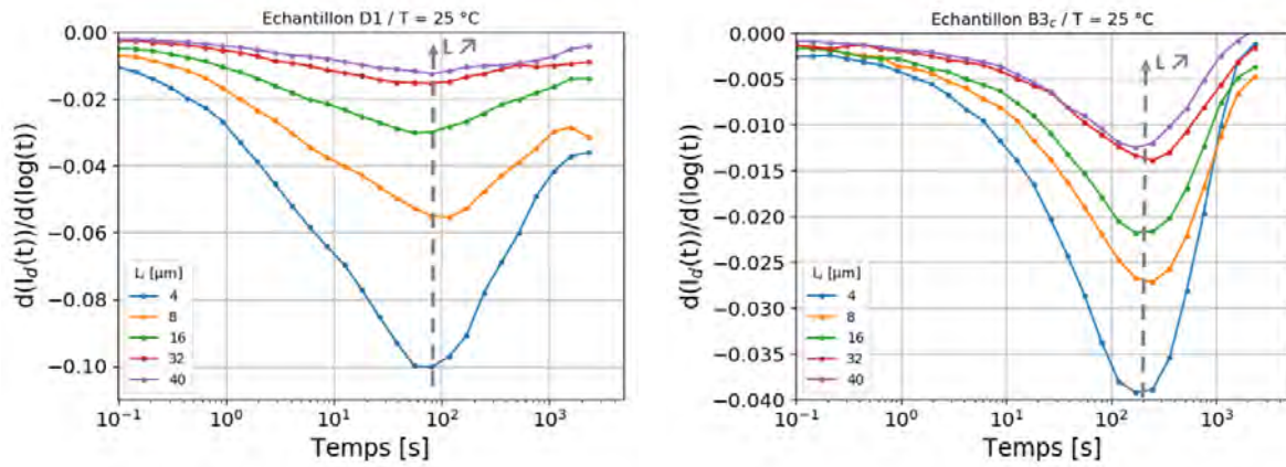
Figure 3.13 Dérivée première dans l'échelle logarithmique temporelle appliquée sur les données de relaxation du courant I_d obtenues, à T = 25^\circ\text{C} , pour différentes distances L_i , avec les échantillons : (a) A1 et (b) B4 b . La ligne en pointillé présente la variation des extremums des creux en fonction de l'augmentation de L_i .
