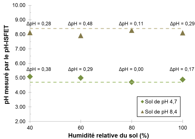
Figure 94 : Comparaison des valeurs de pH mesurées à différents niveaux d'humidité relative dans un sol acide et un sol basique. L'erreur de mesure par rapport à la méthode standard (lignes en pointillé) est indiquée au-dessus de chaque point de mesure
