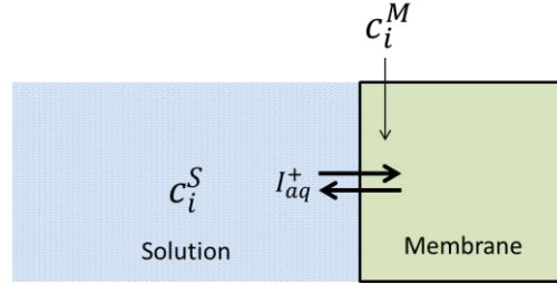
Figure 35 : Interface membrane/solution considérée pour la présentation du modèle PB. La membrane n'est perméable qu'à l'ion I^+
