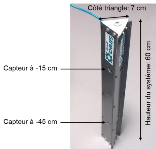
Figure 103 : Photo et dimensions du système
