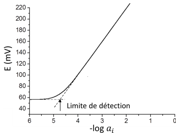
Figure 46 : Définition de la limite de détection d'un capteur potentiométrique
