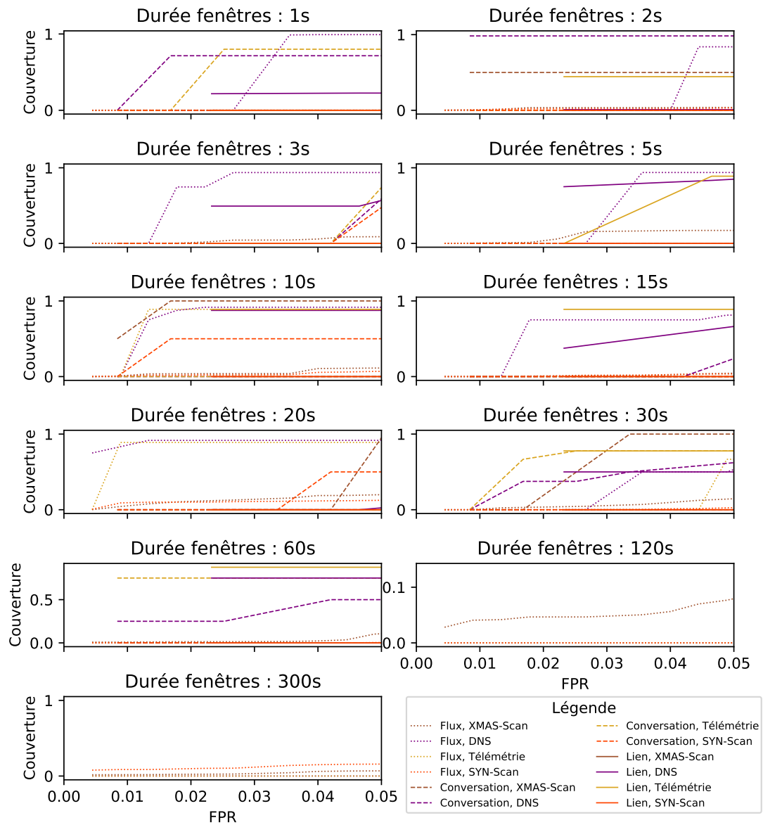
FIGURE 3.18 – Couverture des anomalies par durée des fenêtrés en suivant le score MCC.
