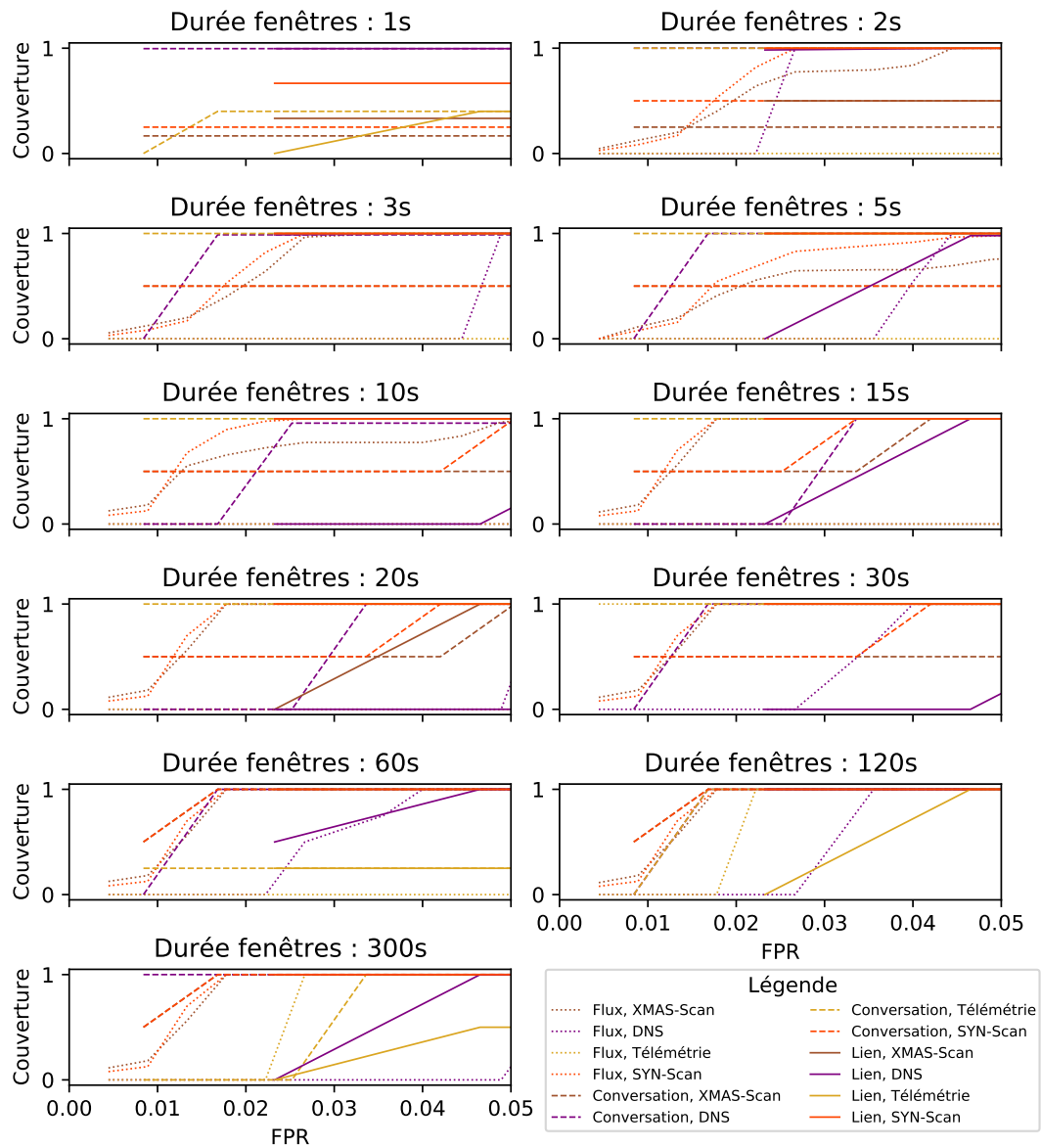
FIGURE 3.23 – Couverture des anomalies par durée des fenêtres en fonction du MCC pour l’algorithme LSTM.
