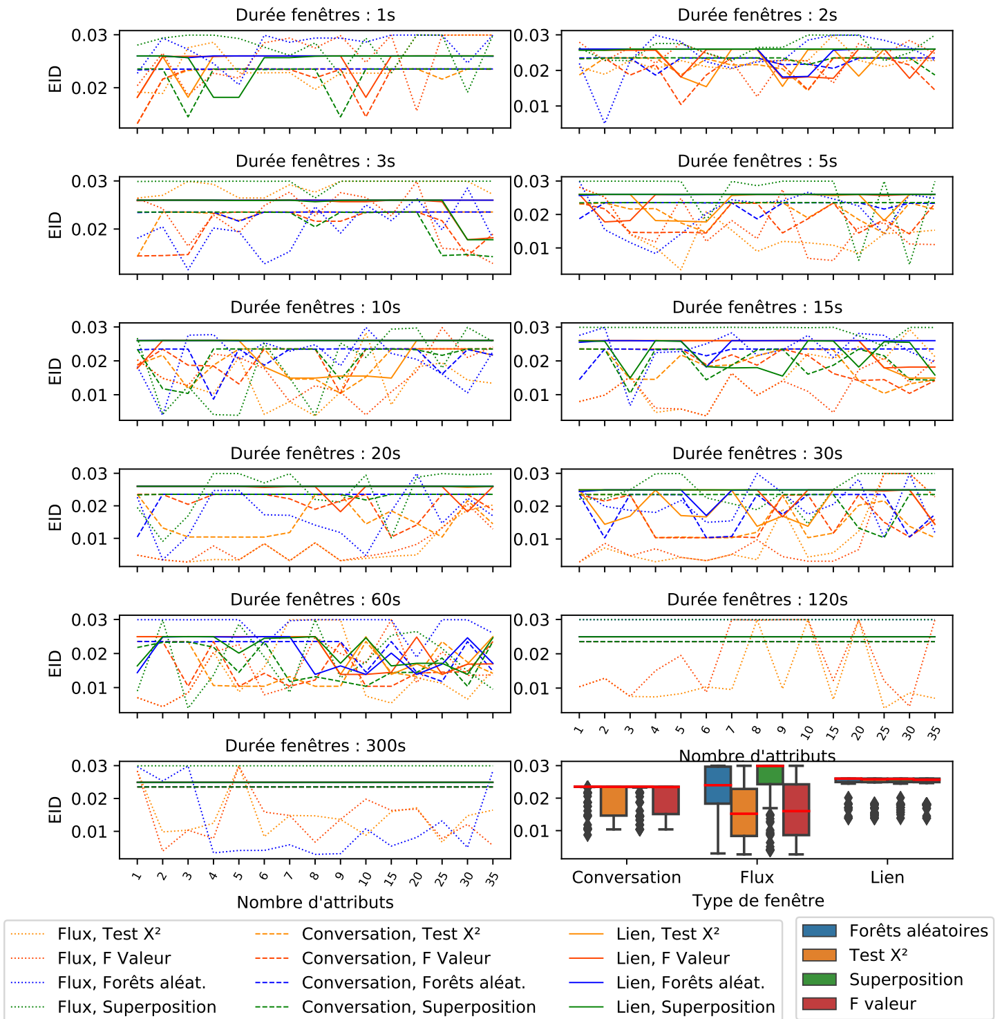
FIGURE 3.16 – Score d’efficacité de la détection (EID) par durée des fenêtres pour l’algorithme HTM.
