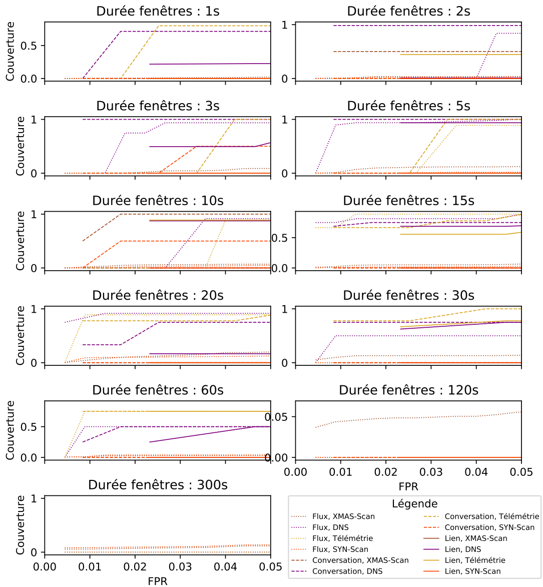
FIGURE 3.19 – Couverture des anomalies par durée des fenêtres selon le score d'efficacité pour l'algorithme HTM.
