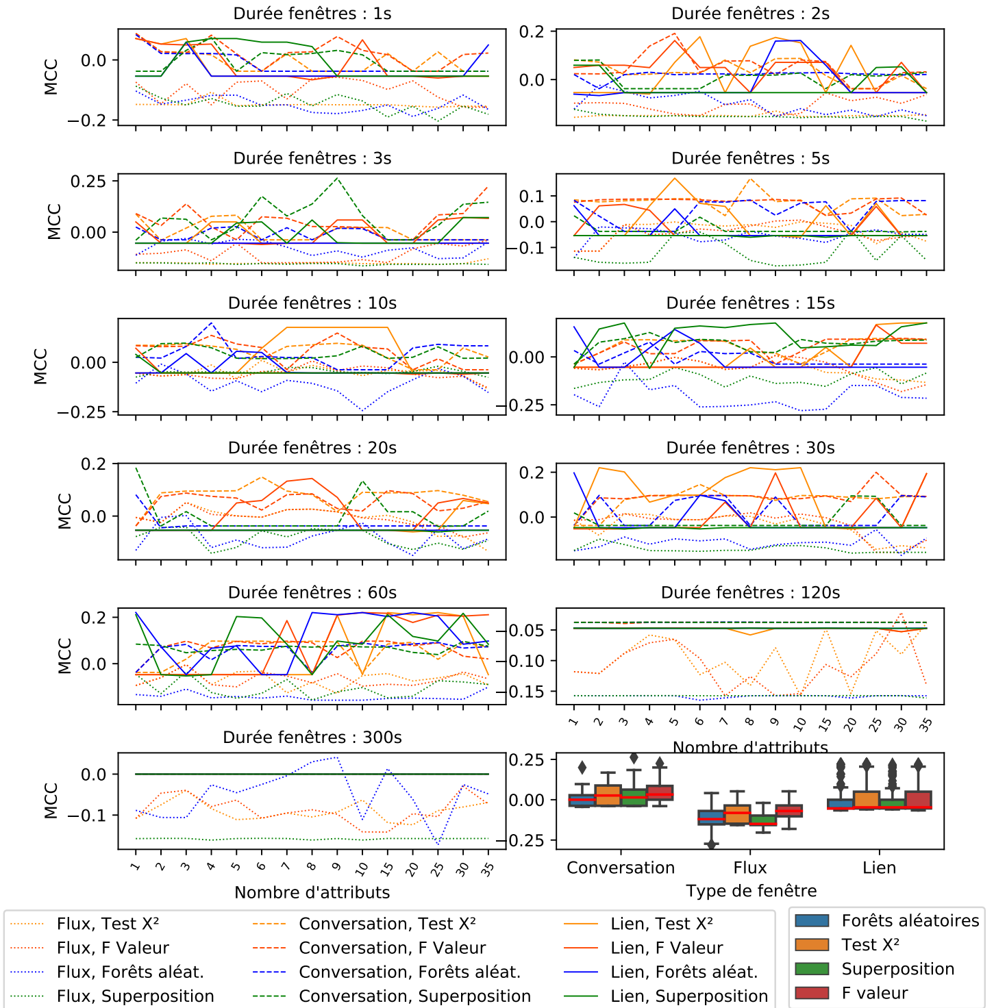
FIGURE 3.17 – Score de MCC par durée des fenêtres pour l’algorithme HTM.
