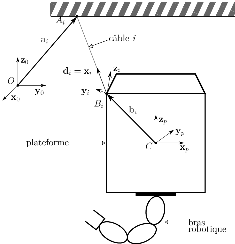
Figure 3.1 – Schéma décrivant les notations pour un RPC
