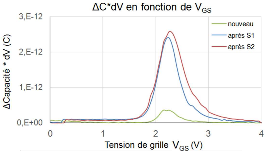
Figure 105 : Intégrale de la capacité par rapport à la tension V_{GS} vieillie à V_{GS} = 4 V
