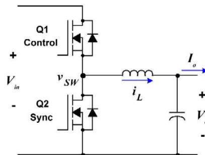
Figure 14 : Schéma d'un convertisseur DC/DC Buck à commutation synchrone
