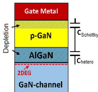
Figure 50 : (a) Modèle équivalent de la capacité de grille dans un HEMT en GaN normalement-off avec la structure p-GaN [66]
