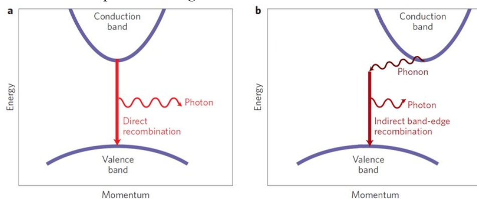
Figure 1 : Structure de bandes d'un semi-conducteur à gap direct (a) et indirect (b)[2]
