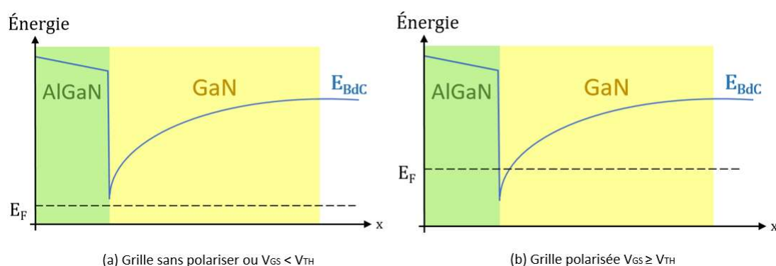
Figure 15 : Diagramme de bandes d'énergie sous la grille d'un HEMT à l'état bloqué(a) et à l'état passant (b)
