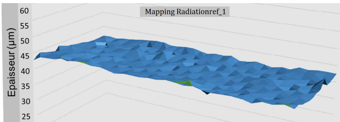
Figure 121 : Mapping de l'épaisseur de la puce Radiationref_1 après amincissement
