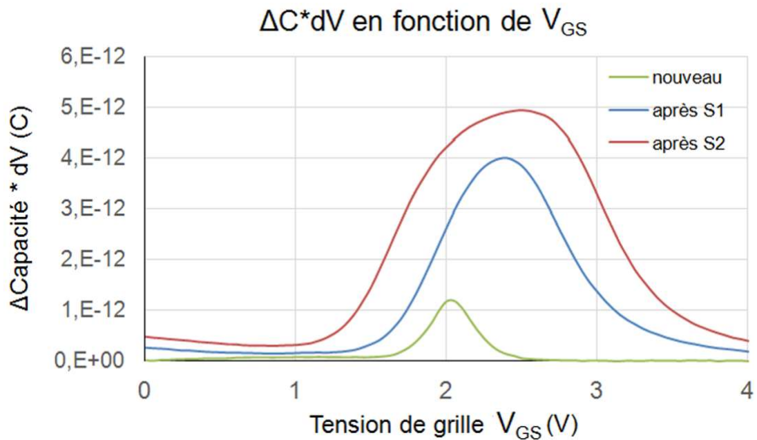
Figure 104 : Intégrale de la capacité par rapport à la tension V_{GS} vieilli a V_{GS} = 5 V
