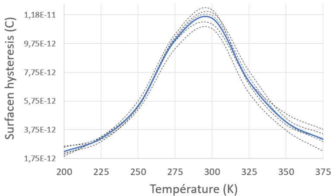
Figure 71 : Surface d'hystérésis (C) en fonction de la température (K). En pointillé les courbes de 5 échantillons, et en bleu la moyenne.
