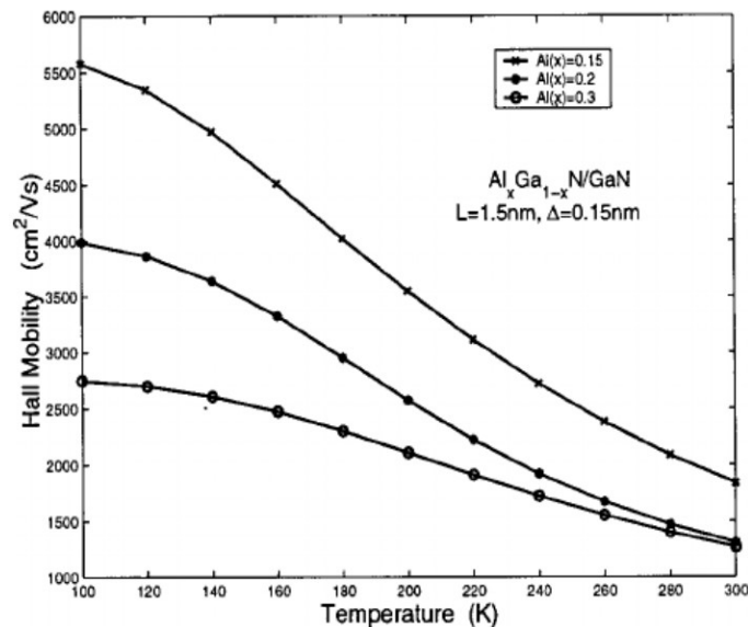
Figure 10 : Mobilité des électrons dans le gaz bidimensionnel en fonction de la température et des différents taux d'aluminium [22]
