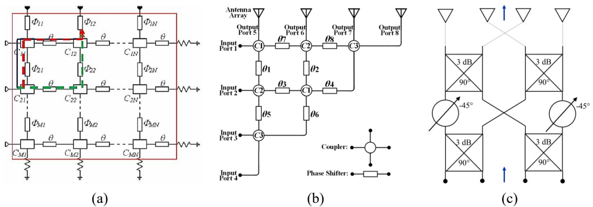
Figure III-3 : Diagramme d'une matrice (a) 3×3 de Blass [17], (b) d'une matrice 4×4 de Nolen [18] et (c) d'une matrice 4×4 de Butler.
