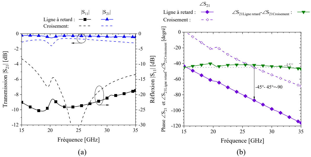
Figure III-23 : (a)-(b) Paramètres S des lignes à retard de la Figure III-21 et du croisement de la Figure III-17 et (b) déphasage entre les lignes et le croisement \angle S_{21 \text{ ligne}} - \angle S_{21 \text{ Croisement}} .
