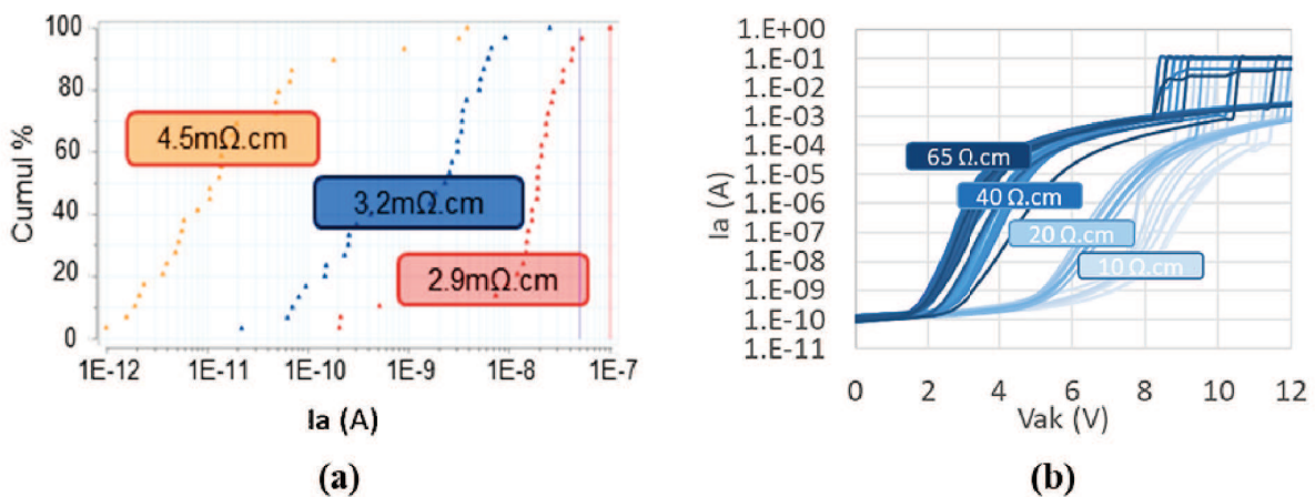
Figure 4.8 : Influence de la résistivité du substrat (a) et de la couche d'épitaxie (b) sur le courant de fuite de la protection
