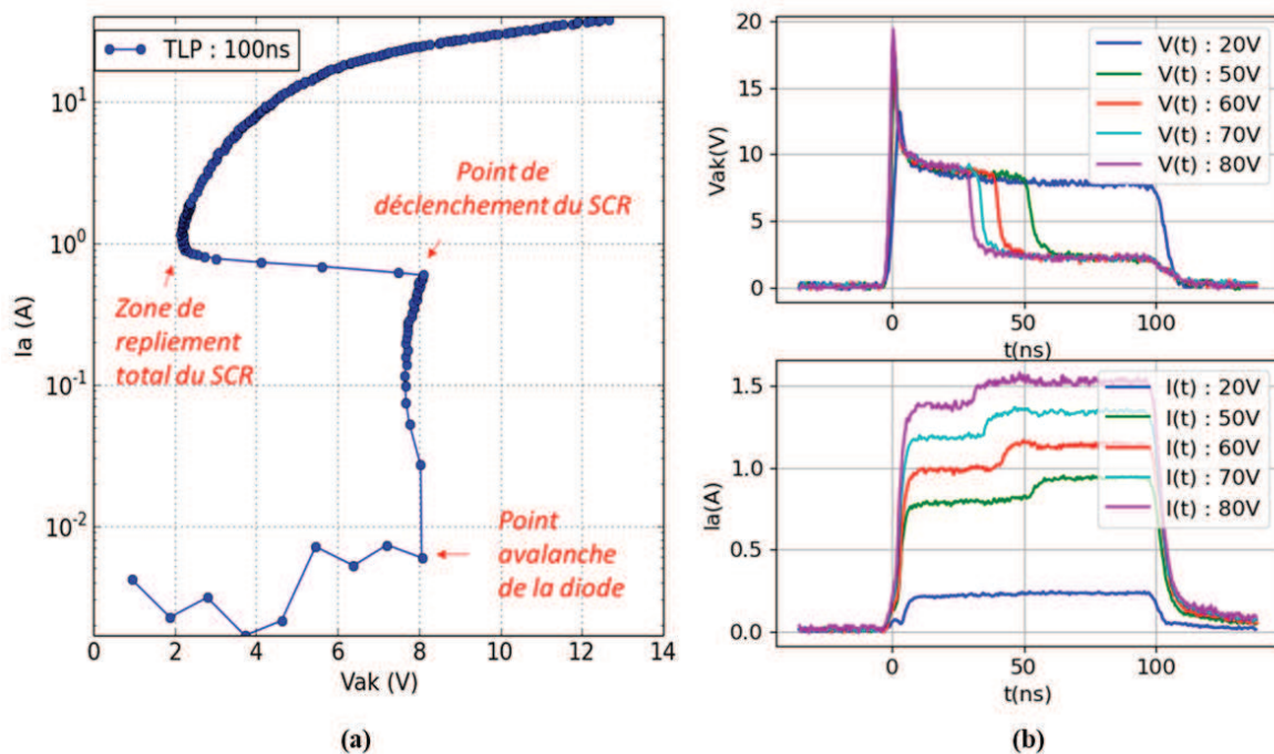
Figure 2.26: Caractéristique I-V de la protection DTSCR (a), et réponses temporelles en courant et en tension pour différents niveaux de précharge TLP (b)
