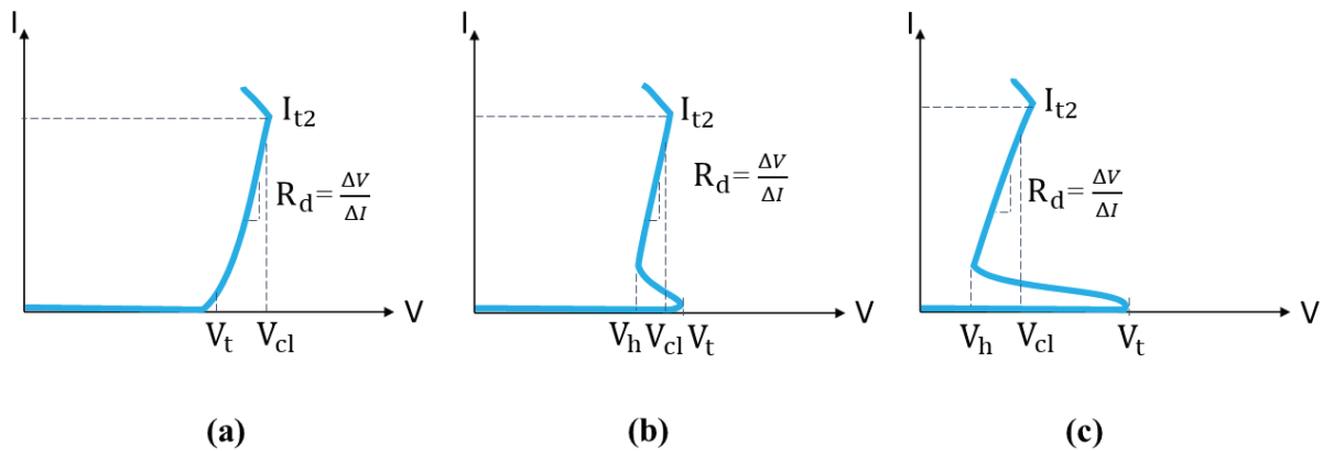
Figure 1.27: Allures typiques des caractéristiques I-V des protections externes : type-diode (a), faible retournement (b) et fort retournement (c) [Adaptée de [INF 19]]
