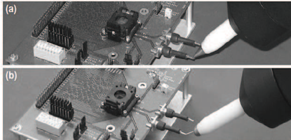
Figure 1.13: Exemple de décharges au pistolet ESD : au contact (a) et dans l'air (b) [VAS 14]
