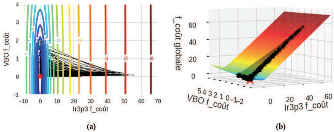
Figure 4.28 : Recherche du minimum (étoile rouge) de la fonction de coût suivi par les courbes de niveaux (a) et de surface (b)
