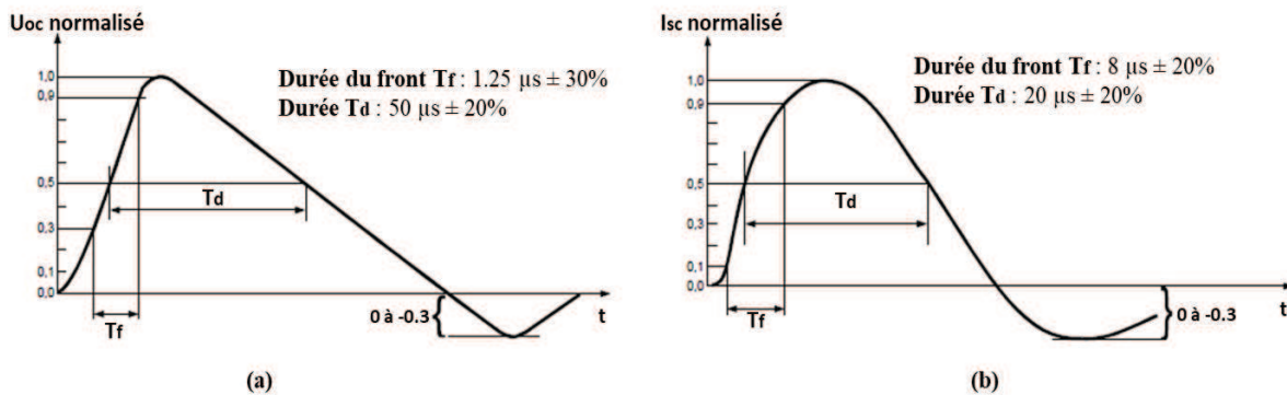
Figure 1.18: Formes d'onde de tension en circuit ouvert ( 1.2/50 \mu\text{s} ) (a), et forme d'onde du courant de court-circuit ( 8/20 \mu\text{s} ) (b) [Adaptée de [IEC 17]]
