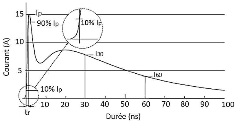
Figure 1.12: Forme d'onde du courant de décharge IEC61000-4-2 au contact à 4 kV dans une impédance équivalente à 2 Ω [Adaptée d'après [IEC 08]]
