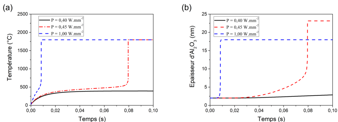
Figure III.4. (a) Evolution temporelle de la température et (b) de l'interface d'alumine d'un nanolaminé soumis à trois densités de puissance différentes ( 0,4 , 0,45 et 1 W.mm -2 ). Le nanolaminé est constitué de 10 bicouches Al/CuO d'épaisseur 300 nm ayant un rapport massique Al:CuO 1:1 et est déposé sur un substrat Kapton ( n=10 , w= 300 nm, \zeta = 1 , d = 2 et \lambda_s=0,1 W.m -1 .°C -1 )
