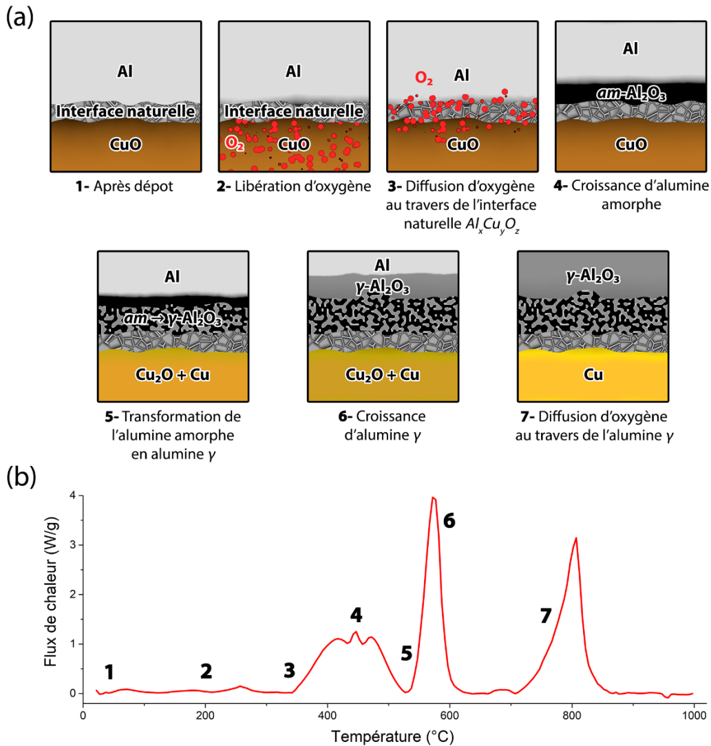
Figure II.13 – (a) Représentation schématique des mécanismes thermiquement activés dans un nanolaminé Al/CuO soumis à une rampe de température. (b) Courbe DSC typique d'un nanolaminé de dix bicouche Al/CuO 2:1 avec une épaisseur de bicouche de 400 nm avec une rampe de température de 10 ^{\circ}C/min . Les chiffres renvoient aux mécanismes correspondants.
