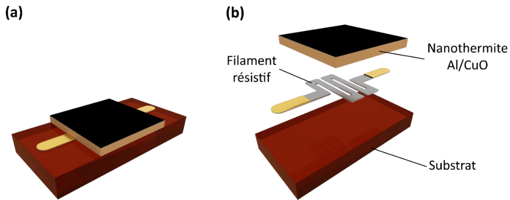
Figure 1.8 - (a) Représentation schématique 3D et (b) vue éclatée d'un pyroMEMS.
