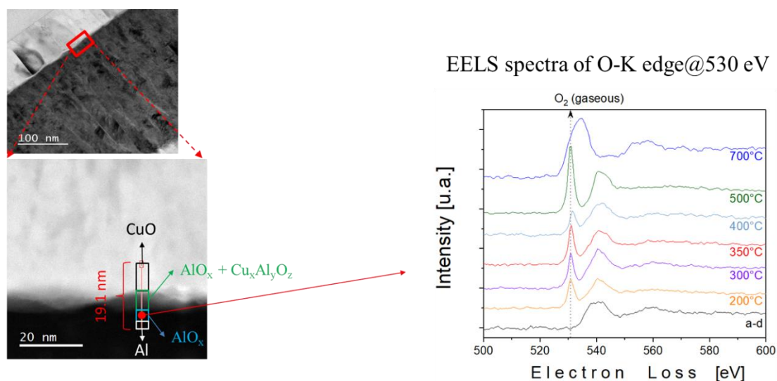
Figure II.11 – spectres EELS O-K-edge 530eV mesuré dans la couche de CuO à 10 nm de Al bottom /CuO interface, après dépôt et chauffé à 100, 200, 300, 350, 500 et 700 °C.
