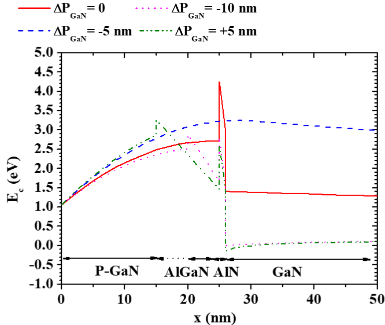
Figure II-7 : Diagramme de bandes pour différentes valeurs de \Delta P_{GaN} à V_{gs} = 0 pour une grille Schottky.
