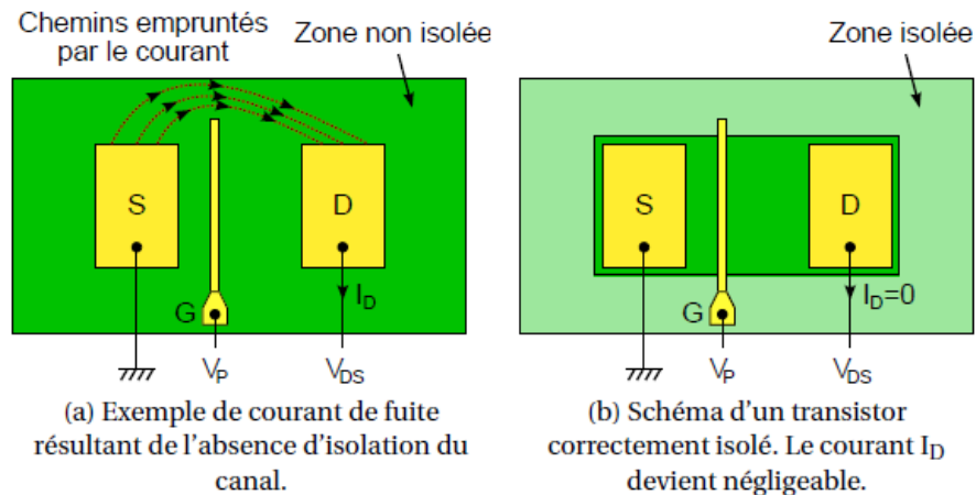
Figure III-48 : Illustration des chemins empruntés par le courants dans le cas d'un transistor polarisé à V_{GS} = V_P dans un cas isolé par MESA et non isolé [9].
