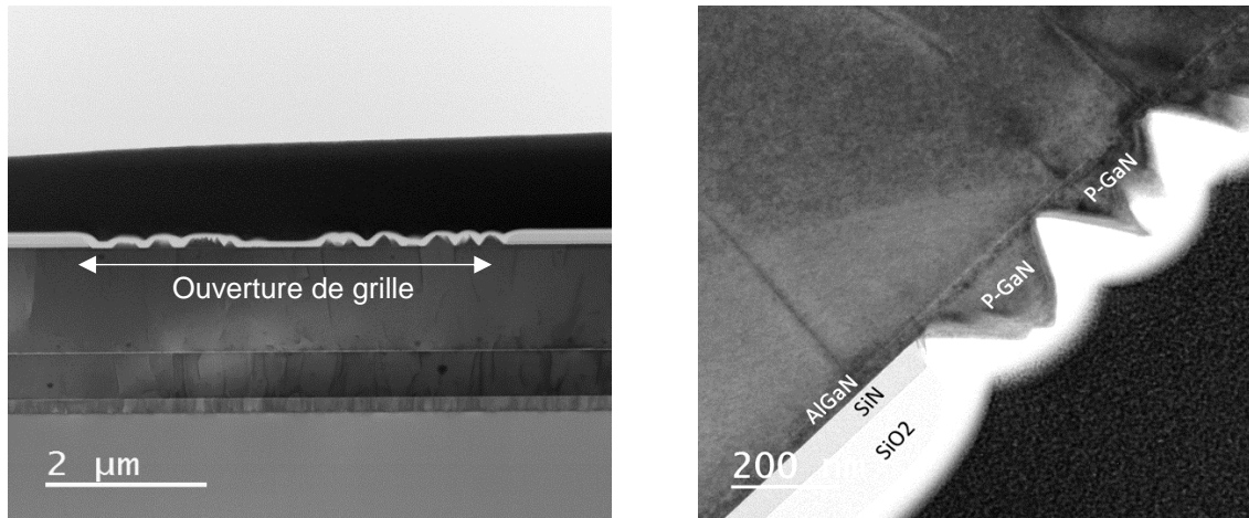
Figure III-31 Coupe TEM d'une reprise d'épitaxie de P-GaN en mode MOCVD de 8 s sur une ouverture de grille de 6 μm.
