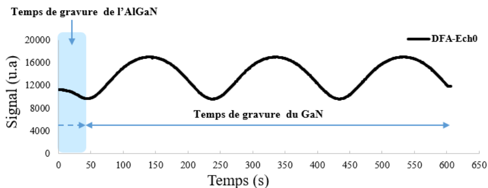
Figure III-17 : Mesures de réflectométrie par interférométrie laser de la gravure RIE par \text{Cl}_2 de l'AlGaN et du GaN.
