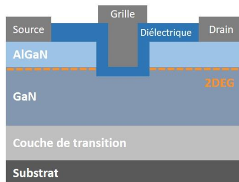
Figure I-13 : Transistor HEMT normally-off avec une grille MIS (Metal Insulator Semiconductor High electron mobility transistor).
