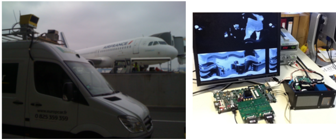
Figure 2.1: Intégration matérielle réalisée dans le cadre du projet SART : à gauche la campagne de mesures réalisée sur l'aéroport de Blagnac avec les capteurs montés sur un camion et à droite le boîtier des caméras VIS/LWIR (long wavelength infrared) et kits de développement sur FPGAs.
