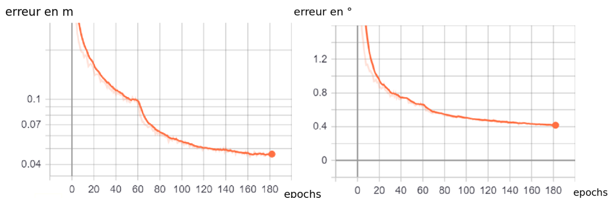
Figure 7-4 - Valeur de la fonction de coût en fonction du nombre d'itération d'entraînement, le nombre d'itération représentant le nombre de fois où le réseau a utilisé l'ensemble des données d'entraînement.
