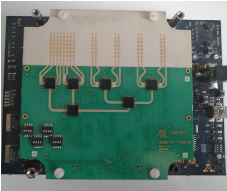
Figure 3-3 - RADAR FMCW fonctionnant à 77 GHz utilisé pour les mesures.
