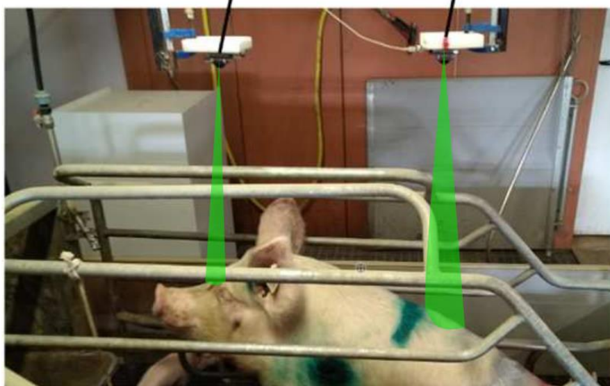
Figure 2-1 - Position de la truie par rapport aux deux RADARs utilisés. Les RADARs étaient séparés de 55cm et placés à 1m40 du sol. En vert est schématisé le faisceau ( 8^\circ d'angle d'ouverture) des deux RADARs.
