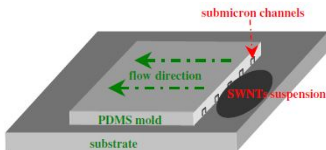
FIGURE 2.4 – Principe de l'alignement par canaux microfluidiques[16] : une suspension de nanotubes de carbone est déposée à droite d'un timbre de PDMS où des microcanaux ont été gravés. Le mouvement du fluide permet l'orientation des nanostructures parallèlement aux canaux.
