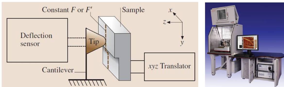
FIGURE 4.2 – A gauche, principe général de l'AFM[27] : la pointe mesure localement la force de l'interaction pointe-échantillon, par la mesure de la déflexion (le plus souvent par la mesure de la position d'un laser par un photodétecteur à quatre cadrans). A droite, l'AFM Icon de Bruker utilisé lors de ces travaux[28]
