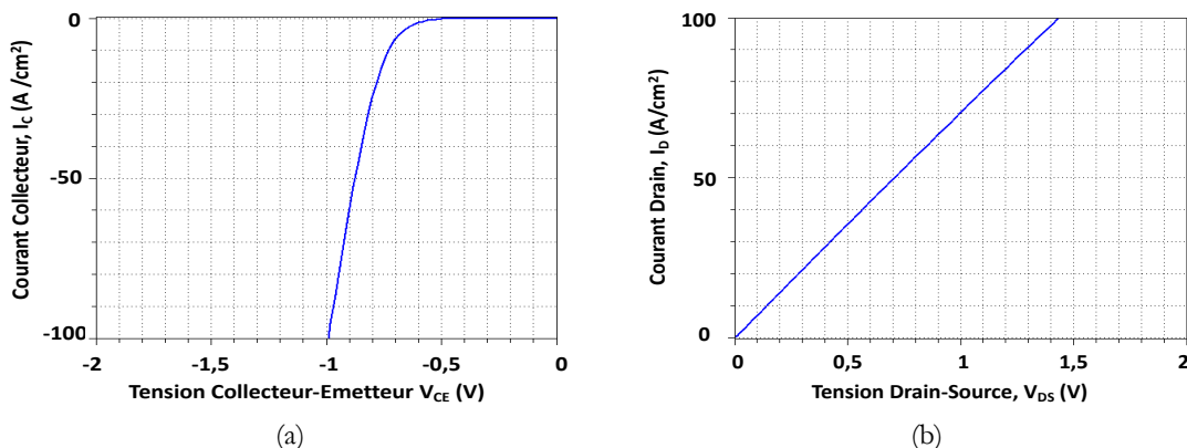
Figure 116 : Caractéristiques I-V à l'état passant des composants P-IGBT (a) et N-VDMOS (b) (tenue en tension : 100\text{ V} ).
