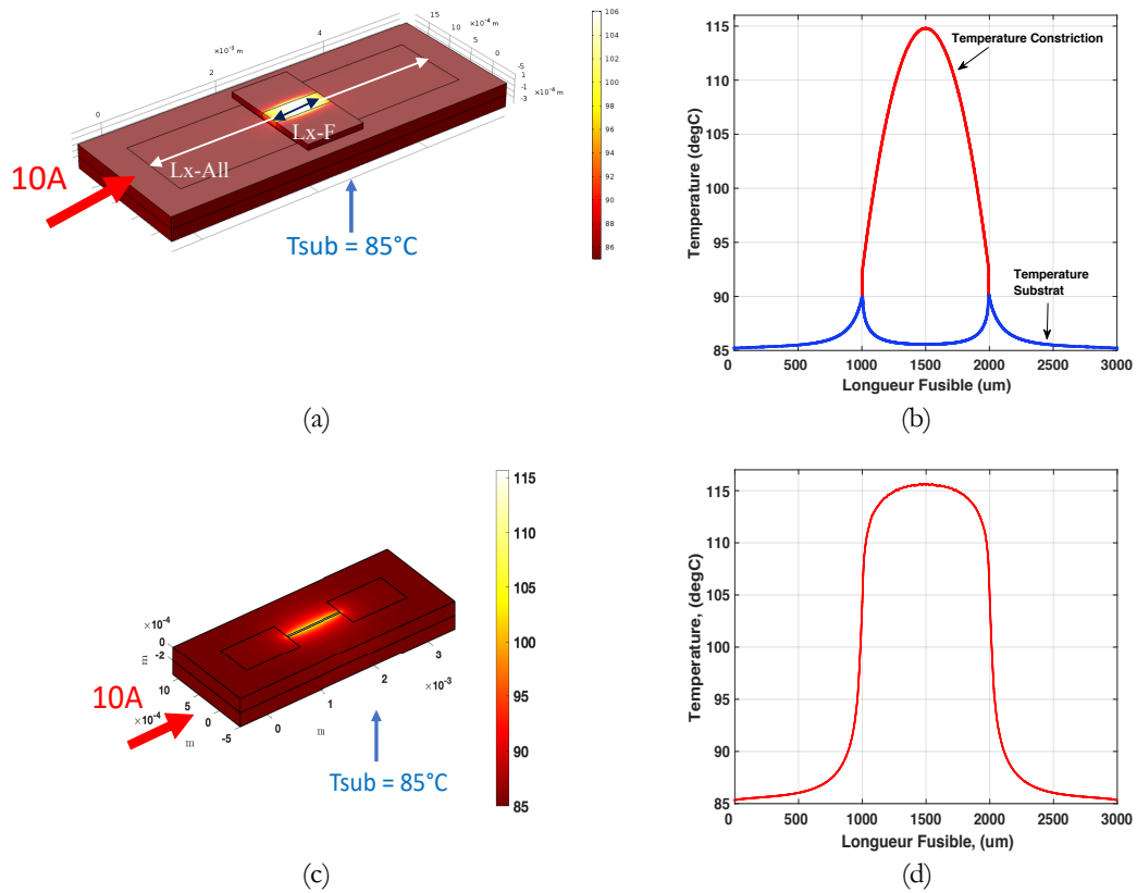
Figure 43 : Cartographie thermique d'un fusible mono-constriction (a) sous 10A/115 °C et le profil thermique associé (b) avec époxy sous la constriction et sans époxy (c-d).
