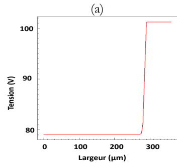
Figure 137 : Distribution des équipotentielles dans la structure montrant les deux composants P-IGBT et N-VDMOS à l'état bloqué.
