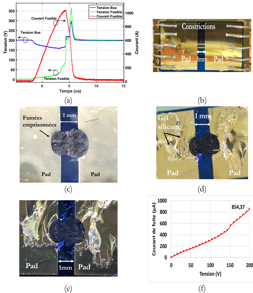
Figure 67 : Résultats du test de claquage à 200V sur une puce fusible à deux constrictions séries (a), photographie de la puce avant claquage (b), après claquage (c), avec un zoom sur la zone constriction droite (d-e) après avoir enlevé le gel, ainsi que les courants de fuites mesurés sous la tension nominale (f) (200 V).
