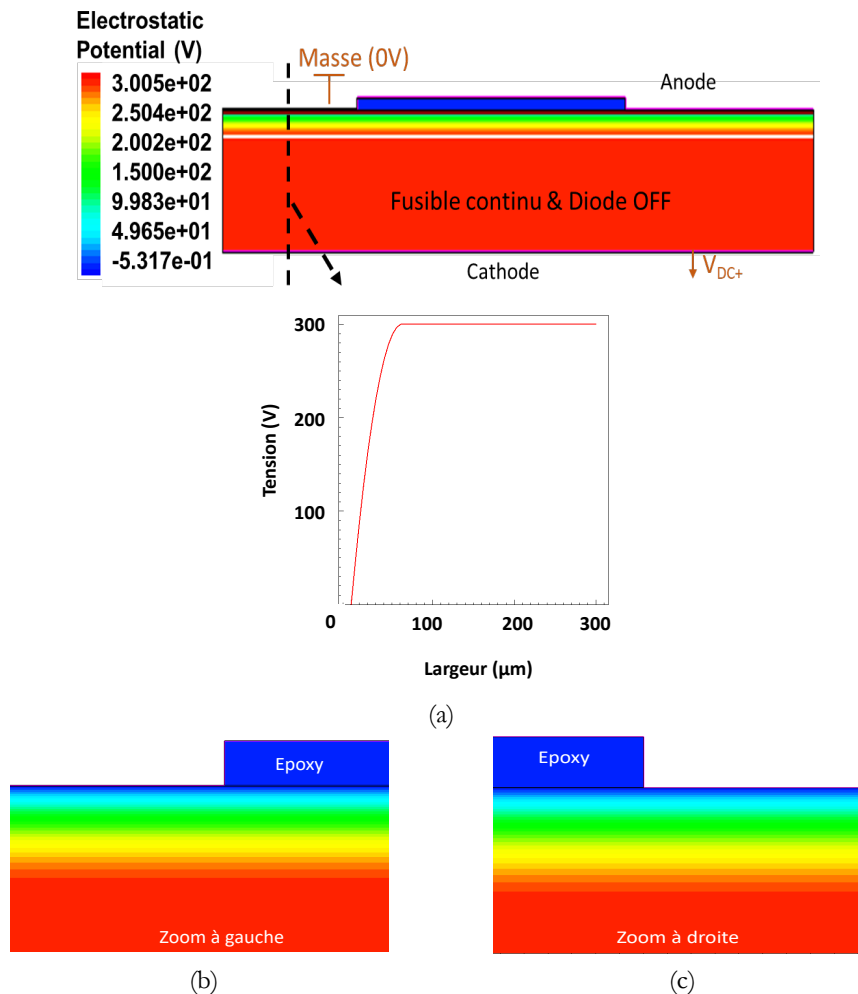
Figure 73 : Distribution des équipotentielles (a) et agrandissements (b et c) autour de la zone époxy.
