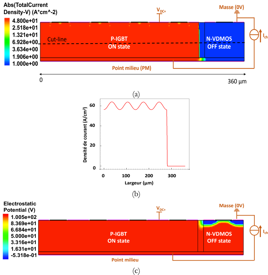
Figure 133 : (a) Distribution de la densité de courant dans l'IGBT à l'état passant, (b) tracé du profil à y=35 \mu\text{m} et équipotentielles montrant la jonction bloquée du N-VDMOS (c) (courant de fuite : 7 \mu\text{A} ).
