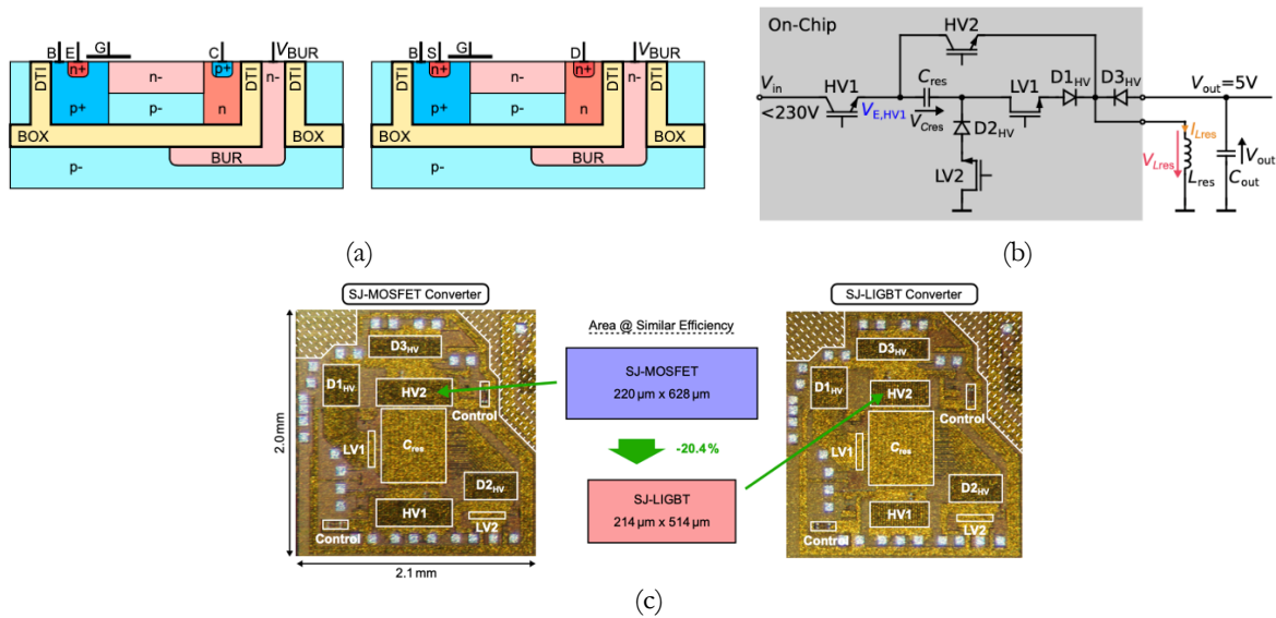
Figure 31 : Architectures SJ-MOSFET et SJ-LIGBT (a), circuit convertisseur de test (b) et intégration du circuit intégré (c).
