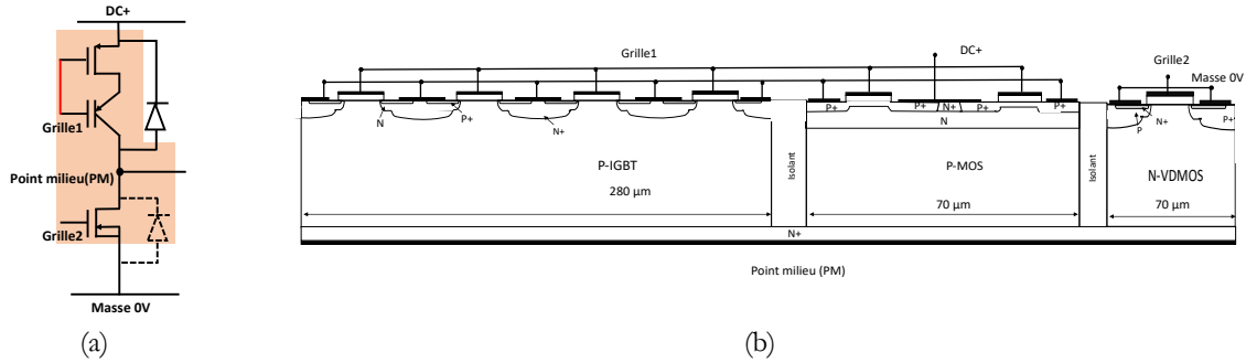
Figure 164 : Circuit électrique et structure monolithique associée du bras P-IGBT, P-MOS et N-VDMOS.
