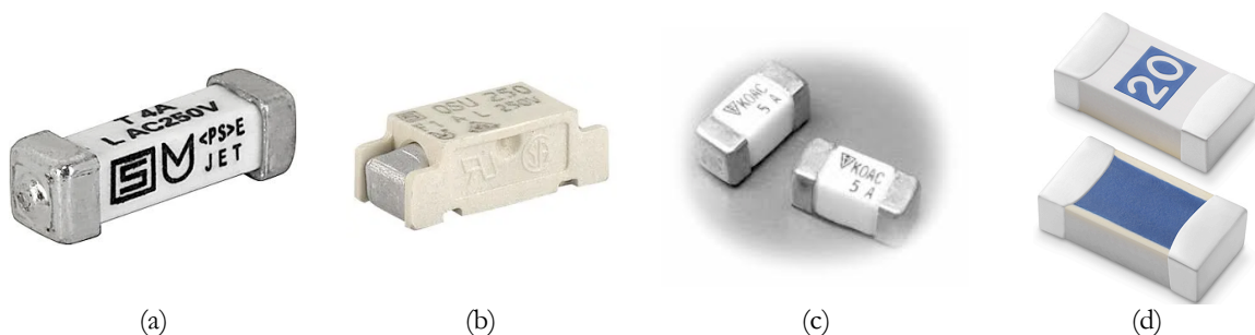
Figure 10 : Exemples de quelques fusibles CMS : (a) Schurter OSU 250 [17], (b) Schurter UMT 250 [18], (c) KOA CCF1N5 [19] et (d) Littelfuse 501 series [20].
