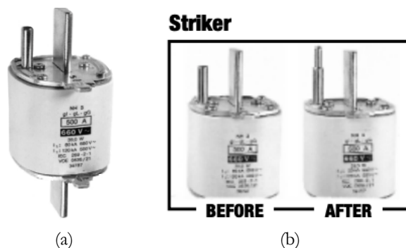
Figure 8 : Exemples de fusibles avec déclencheur (percuteur) : Ferraz Schawmut 690 V/500 A [14].
