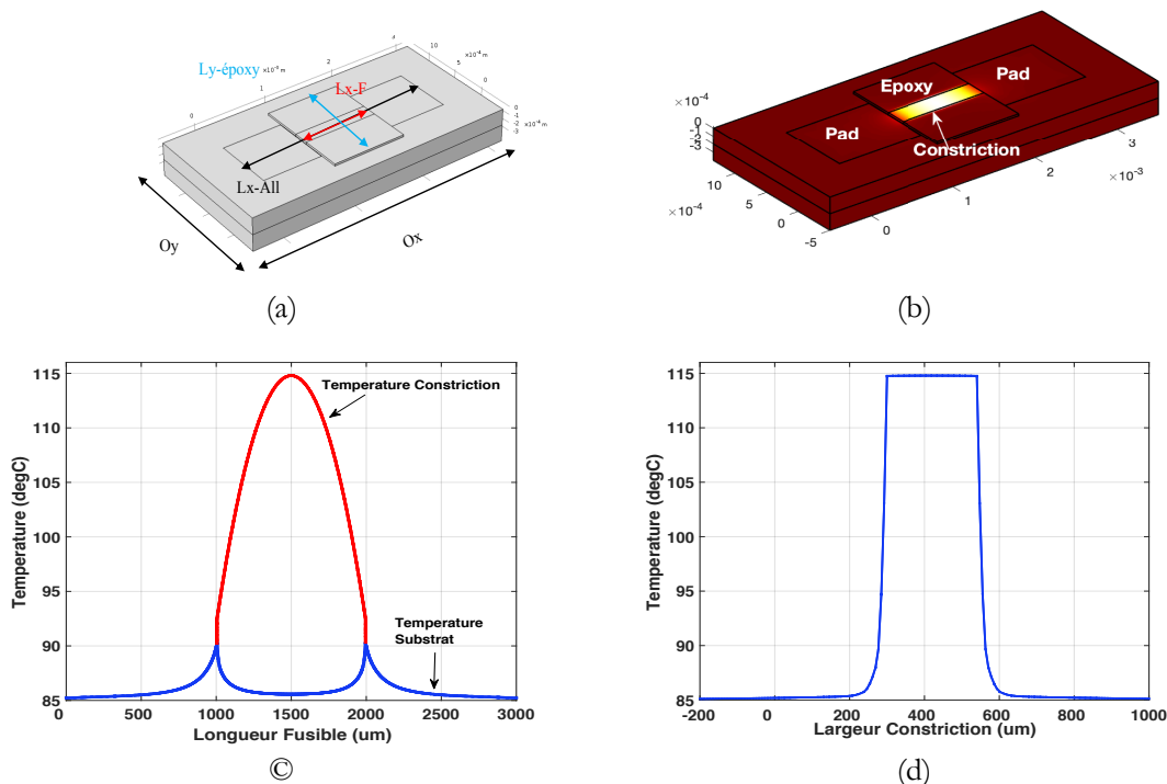
Figure 46 : Géométrie d'un fusible mono-constriction (a), sa cartographie thermique pour 10 A – 115 ^{\circ}\text{C} (b), le profil thermique en longueur du fusible (c) ainsi que le profil thermique en largeur de la constriction (d).
