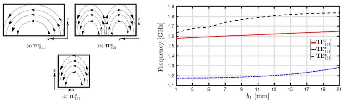
Figure IV.34 Fréquences de résonance des modes TE_{\delta 11}^x , TE_{1\delta 1}^y et TE_{\delta 12}^x . en fonction de b_1 pour d_1 = 15\text{mm} ; w_1 = 15\text{mm} ; \epsilon_{\text{hole}} = 1
