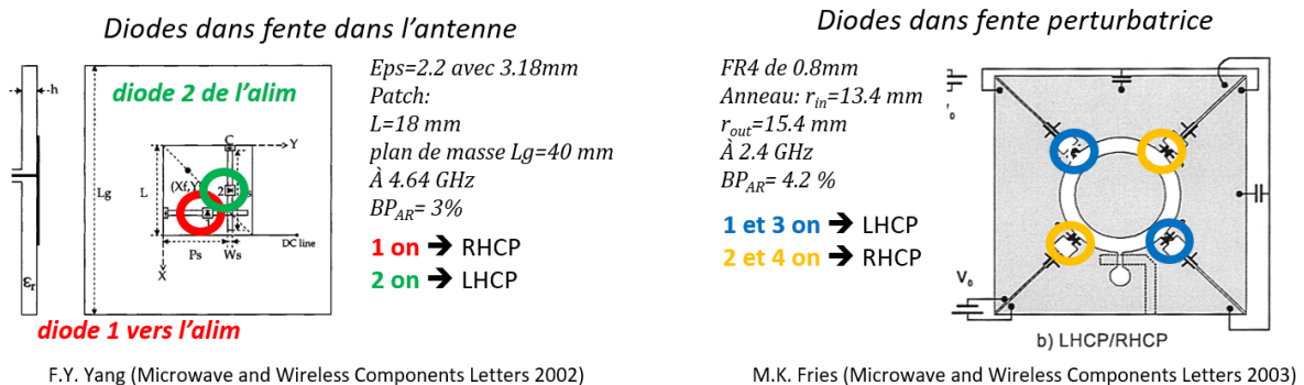
Figure I.1: Antennes à commutation de polarisation circulaire avec diodes insérées dans l'antenne ou dans la fente
