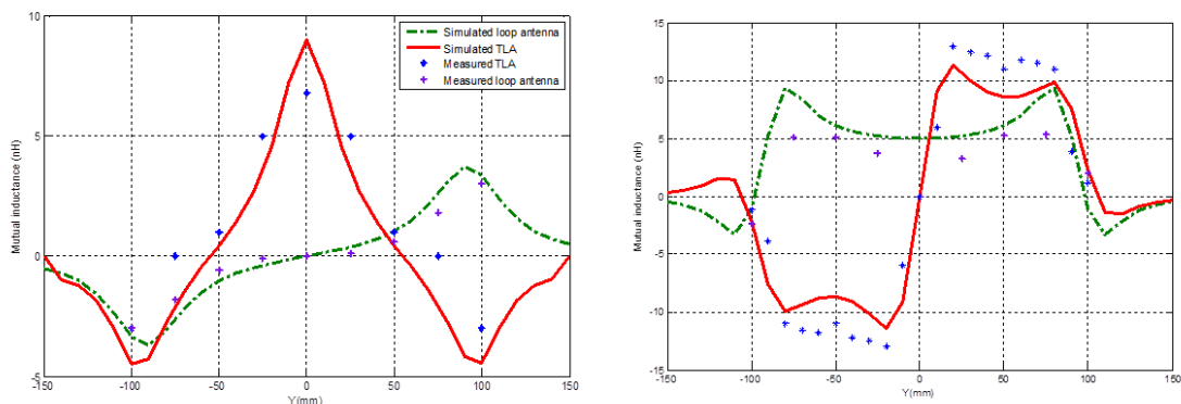
Figure III.10 Inductance mutuelle entre l'antenne lecteur (TLA ou rectangulaire) et TAG (30mm de diamètre) pour les configurations perpendiculaire (à gauche) et parallèle (à droite)
