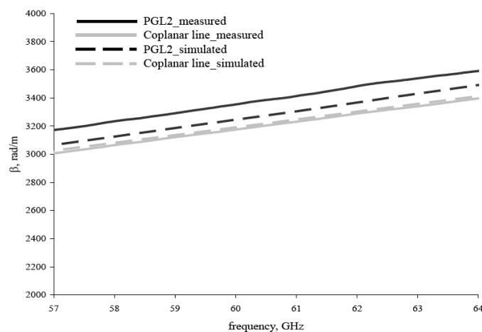
Figure II.11: Constante de phase \beta (rad/m) mesurée et simulée de la PGL (PGL2) et de la ligne coplanaire en fonction de la fréquence (57-64GHz).
