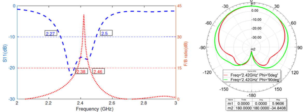
Figure IV.40 Adaptation (en bleu à gauche), rapport du rayonnement arrière sur avant (en rouge à gauche), diagrammes de rayonnement (à droite)
