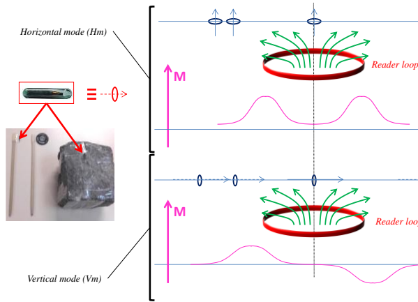
Figure III.21: Tag en verre dans les galets (en haut à gauche) dans les modes horizontaux (Hm) et verticaux (Vm) avec l'inductance mutuelle quand le tag est petit
