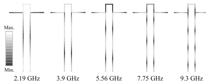
Figure I.3: Distribution du champ électrique dans la ligne coplanaire avec une fente perpendiculaire (sans patch)
