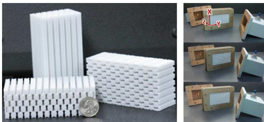
Figure IV.41 a) Matériaux diélectriques anisotropiques b) sous test [GAR 12]
