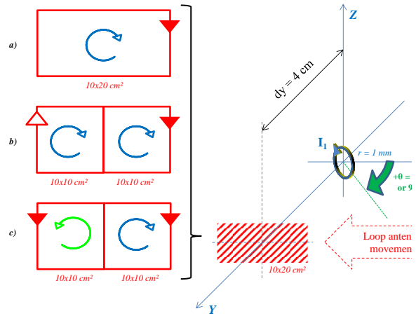
Figure III.22: Surface de la boucle lecteur et dipole magnétique équivalent au tag en verre. Représentation des 3 différentes solutions étudiées
