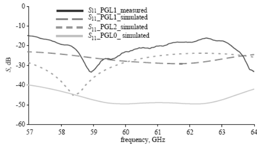
Figure II.12: Simulation et mesure du paramètre de réflexion de la transition (pour une largeur de ligne de 100\mu\text{m} et de fentes 75\mu\text{m} pour la ligne coplanaire)
