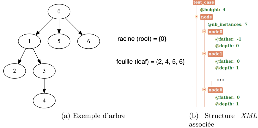
FIGURE 6.10 – Exemple d'arbre.
