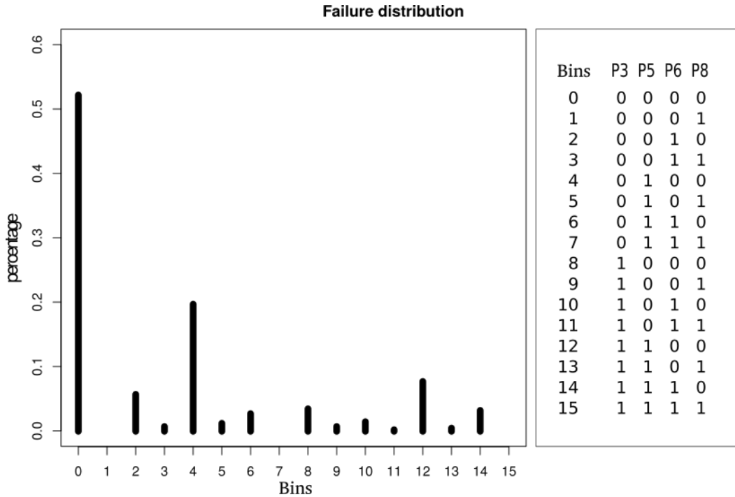
FIGURE 3.4 – Fréquence relative des violations de propriété évaluée sur les 400 exécutions ( X_{80,5} ).
