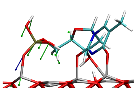
b) Déformation de F due au déplacement de 1,50 Å de OP1
