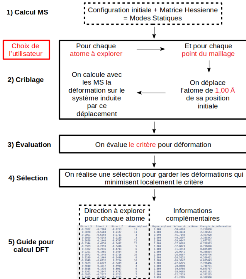
FIGURE 1.7 – Logigramme du processus de sélection des MS. En rouge, apparaissent les paramètres définis par l'utilisateur : la liste des atomes à explorer, le maillage, le rayon de criblage et le critère utilisé. Les résultats du criblage sont résumés à l'étape 5 sous la forme d'un récapitulatif des directions à explorer. Ce fichier récapitulatif sera présenté en détails dans la partie 1.5.
