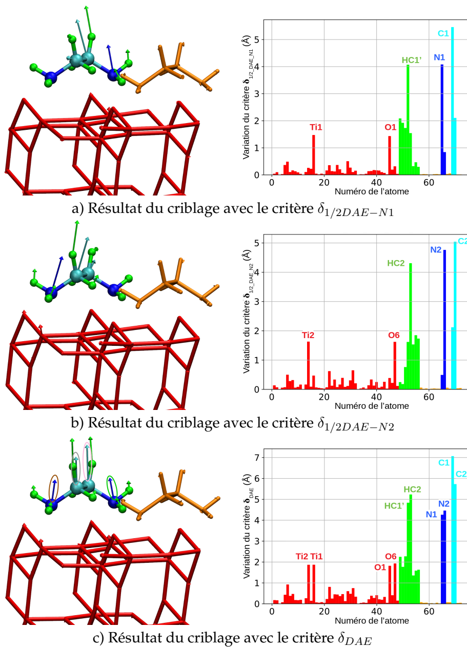
FIGURE 1.15 – Criblages réalisés sur le système BrBr avec différents critères : a) critère \delta_{1/2DAE-N1} , b) \delta_{1/2DAE-N2} et c) \delta_{DAE} . Pour chaque critère est représenté à gauche les directions optimisées sur chaque atome et à droite le graphique montrant l’influence de l’atome sur la valeur du critère. Les atomes de la surface sont colorés en rouge, ceux de la DAE2 en orange, les atomes d’hydrogène de la DAE1 sont en vert, les atomes de carbone en bleu et les atomes d’azote en cyan. Les directions entourées seront étudiées, le code couleur est celui de la figure 1.13.
