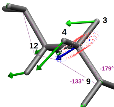
FIGURE 1.9 – Répartition du maillage de la sphère lorsque l'on pondère par l'énergie de la déformation, ici représentée sur l'atome 11. On remarque que l'atome peut difficilement se déplacer vers les atomes à proximité (atomes 12, 9, 3 et 4).
