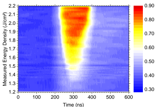
Figure 4. Cartographie TRR obtenue pour une couche de Si 0.6 Ge 0.4 .
