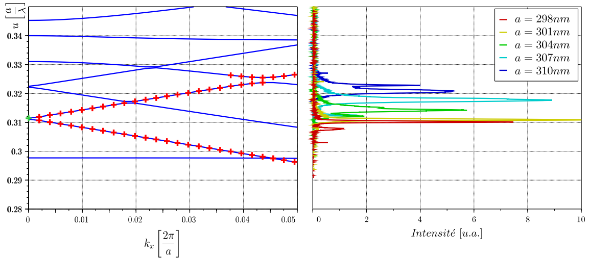
FIGURE 4.29 – Gauche : diagramme de bandes (calcul MPB) d'un guide W3 optimisé. les croix rouges indiquent la dispersion du mode guidé fondamental. La croix verte le point de fonctionnement DFB en \Gamma . Droite : spectres d'émission laser expérimentaux pour différents paramètres de maille.
