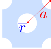
FIGURE 3.9 – Cristal photonique en maille diamant : en rouge le paramètre de maille a ; en bleu le rayon des trous r , en unités de a .
