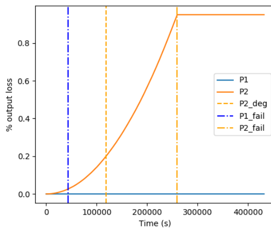
FIGURE 5.7 – Évolution de la dégradation pour chaque panneau jusqu'à la défaillance
