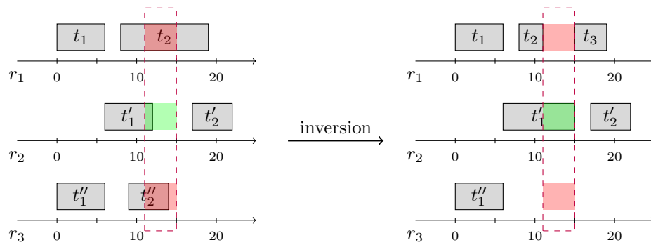
FIGURE 2.14 – Exemple de mouvement de 3-inversion sur un petit intervalle.
