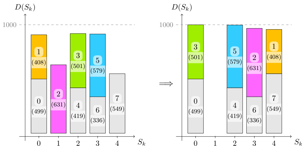
FIGURE 4.8 – Solution initiale (gauche) et solution obtenue après le mouvement \mathcal{M}_{chain} version « déplacements horizontaux » (droite)
