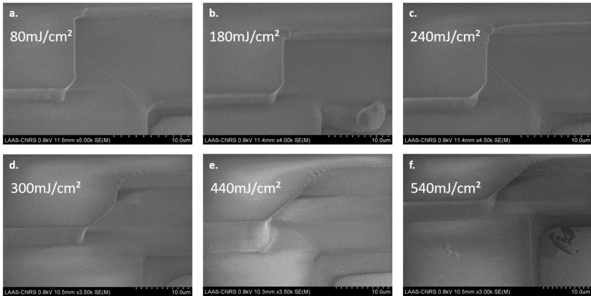
Figure 9 : Caractérisation par MEB des différentes doses d'insolation et de l'épaisseur de la NLOF sur les flancs inversés. a), b) et c) photos de la NLOF de 5\mu\text{m} d'épaisseur et d), e) et f) de la NLOF de 10\mu\text{m} d'épaisseur avec la dose respective indiquée sur chacune des photos.
