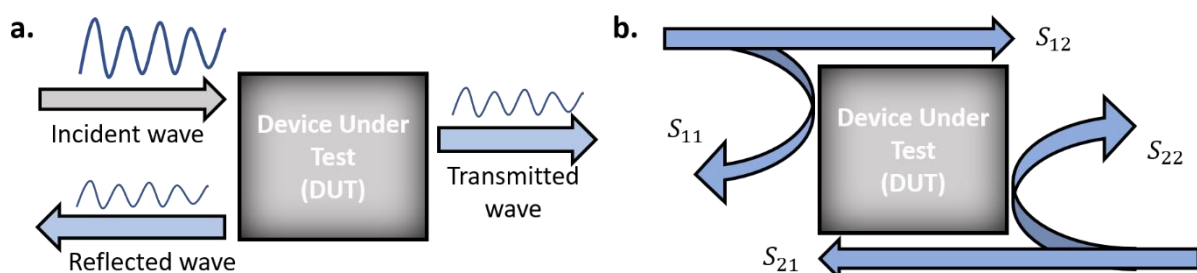
Figure 10 : (a) Principe de transmission et de réflexion des ondes hyperfréquences. (b) Traduction en termes de paramètres S.
