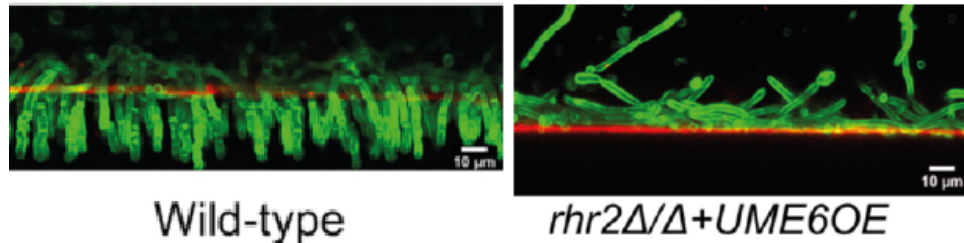
FIGURE 1.32 – Le mutant de la voie de synthèse de glycérol rhr2\Delta/\Delta + UME6^{OE} produit des hyphes mais est incapable d'envahir le gel de polyacrylamide (module d'Young 650 kPa). Notons la surexpression du facteur de transcription UME6 , qui permet de retrouver l'expression des adhésines ALS3 et HWP1 , fortement diminuées chez le mutant rhr2\Delta/\Delta [79]
