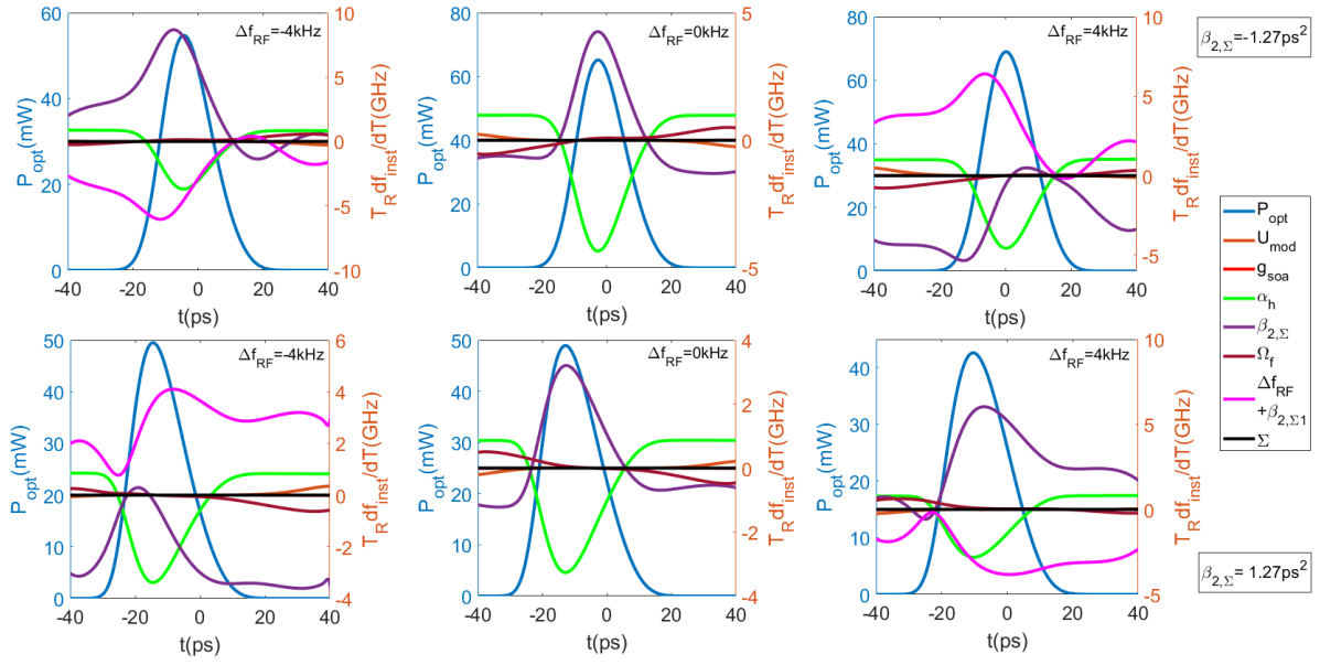
FIGURE 3.19 – Contributions des composants optiques à la fréquences instantanées des impulsions optiques à l'état stationnaire. Les dispersions intra-cavité considérées sont de \pm 1.27 ps^2 , pour trois valeurs de detuning différents \Delta f_{RF} \in \{-4, 0, 4\} ps . La composante linéaire du chirp induit par dispersion chromatique compense celle du front montant imposée par SPM pour \beta_{2,\Sigma} < 0 et descendant pour \beta_{2,\Sigma} > 0 sous condition de parfaite synchronisation du COEO (obtenues respectivement pour \Delta f_{RF} = 4 kHz et \Delta f_{RF} = -4 kHz ).
