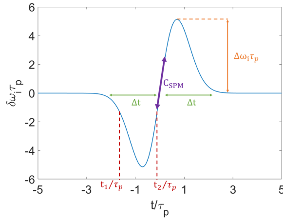
FIGURE 2.18 – Profil de fréquence instantanée d'une impulsion gaussienne non chirpée et modulée en phase par SPM. Le chirm imposé par SPM ( C_{SPM} ) est donné par la dérivée de \delta\omega_i autour du maximum d'intensité ( t/\tau_p \in [-1, 1] ). L'amplitude de modulation de fréquence \Delta\omega_i pour un profil impulsionnel donné, détermine l'intervalle \Delta t sur lequel une même valeur \delta\omega_i est atteinte pour deux instants t distincts, donnant lieu à une figure d'interférence visible sur le spectre optique associé.
