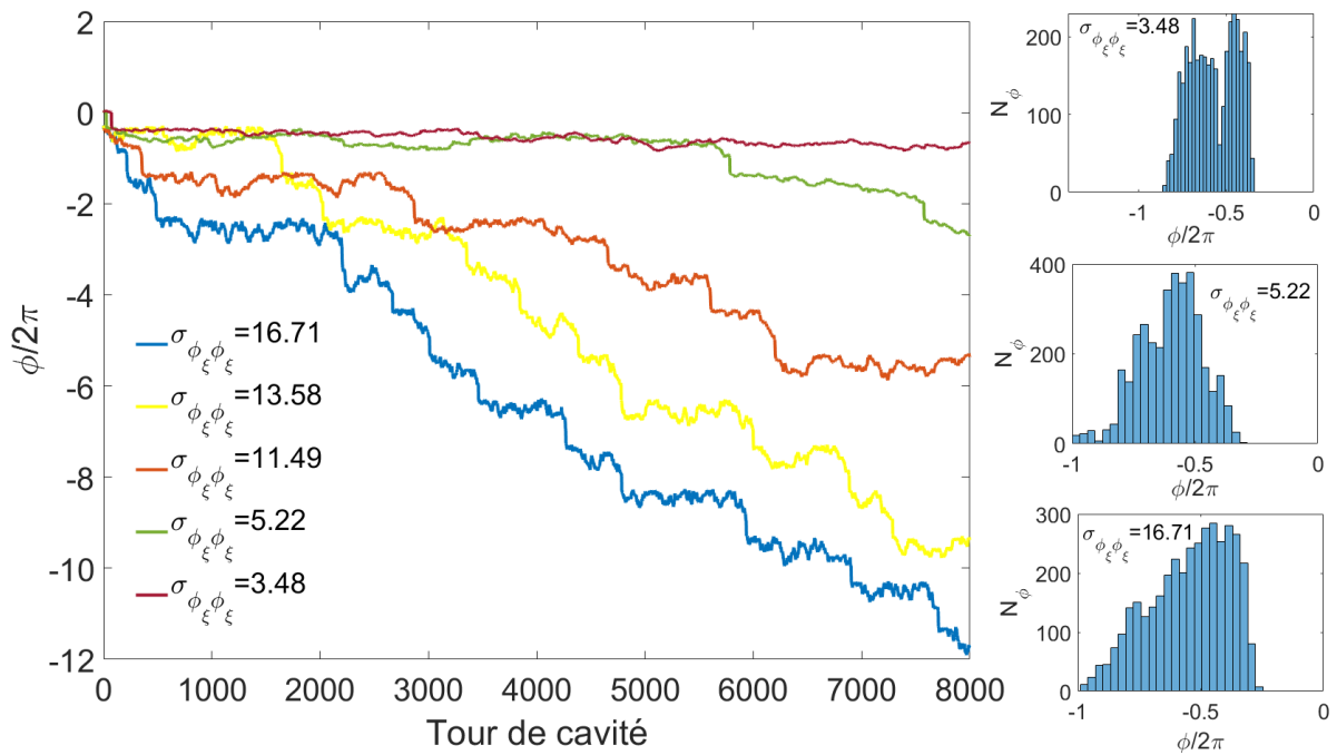
FIGURE 3.28 – Dérive de \phi_\xi calculé à partir de (3.68) soumis à une stimulation en bruit gaussien d'écart-type \sigma_{\phi_\xi\phi_\xi} (rad) dans le cas d'un COEO avec filtre optique, nous permettant de passer d'un système à deux dimensions (eq.3.68 et eq.3.69) vers un problème à une dimension (eq.3.68). La dérive s'accroît avec la variance du bruit considéré. Les histogrammes présentés sur la colonne de droite donnent la répartition de \phi_\xi associée aux courbes présentées sur la figure de gauche. La répartition favorise un angle négatif moyen du fait de la pente de potentiel [18]-[20].
