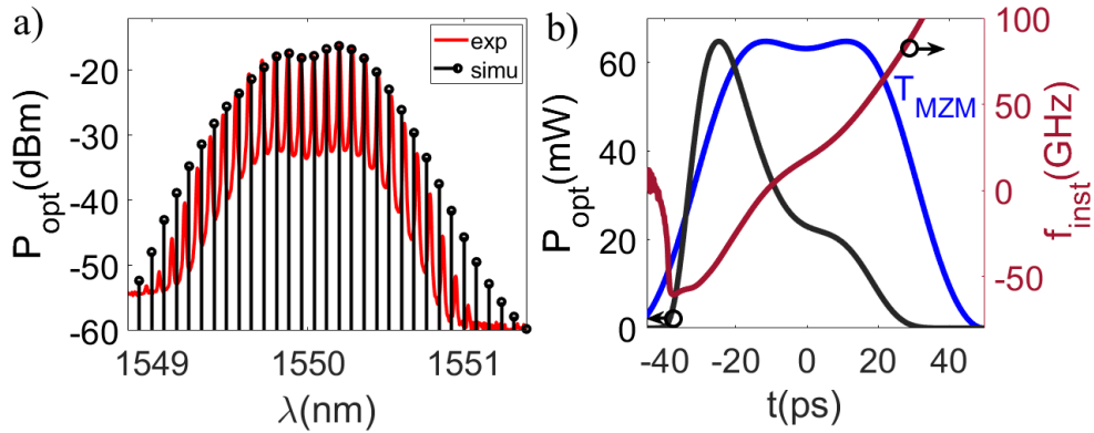
FIGURE 5.11 – a) Spectre optique symétrique simulé du COEO pour une dispersion intra-cavité \beta_{2,\Sigma} = 10.16 \text{ ps}^2 et pour un detuning à la limite de la bande de verrouillage \Delta f_{RF} = -12 \text{ kHz} . Le spectre optique expérimental (en rouge) a été obtenu avec CFBG ( \beta_{2,\Sigma|exp} = 0.5 \text{ ps}^2 ). Le spectre expérimental a été décalé en longueur d'onde et en puissance de sorte à comparer sa forme spectrale avec celle obtenue par simulation. La différence d'ISL entre les deux spectres est due à l'utilisation d'un résonateur RF centré sur 10.29 \text{ GHz} , par rapport aux 10 \text{ GHz} considérés par simulation. b) Profil impulsionnel associé au spectre simulé auquel est ajouté le profil de modulation du MZM (normalisé par rapport au profil d'intensité optique).
