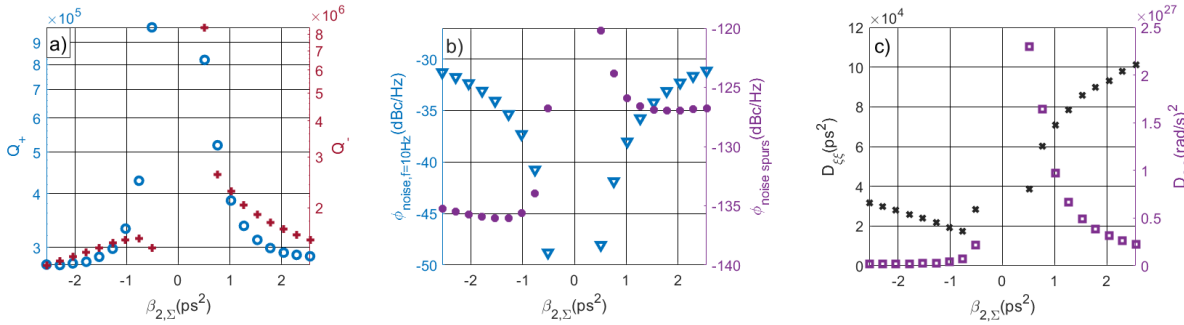
FIGURE 4.12 – a) Évolution des facteurs de qualité Q_+ et Q_- , b) du bruit de phase proche porteuse ( \phi_{noise, f=10Hz} ) et de l’amplitude des pics de corrélation de bruit ( \phi_{noise spurs} ), c) des coefficients de diffusion D_{\xi\xi} , D_{\Omega\Omega} suivant \beta_{2,\Sigma} .
