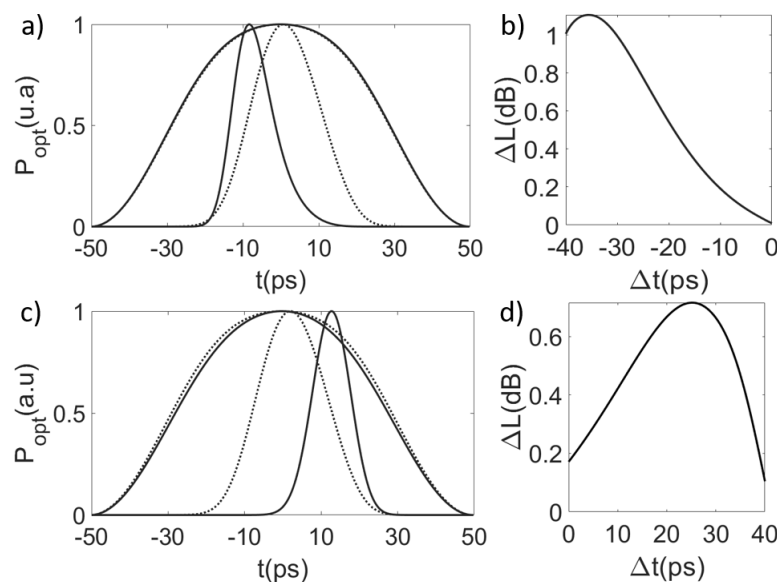
FIGURE 3.36 – a) Profil impulsionnel normalisé du COEO simulé pour un detuning nul ( \Delta f_{RF} = 0 ) et une dispersion chromatique \beta_{2,\Sigma} = -2.55 ps^2 (courbe en pointillés) et \beta_{2,\Sigma} = -0.51 ps^2 (courbe pleine). Les portes de modulation du MZM associées à chacune des valeurs de \beta_{2,\Sigma} sont aussi affichées (avec pour maximum de transmission T_{mzm} = 1 ). b) Différence de pertes \Delta L = L_{\beta_{2,\Sigma}=-2.55} - L_{\beta_{2,\Sigma}=-0.51} lorsque la position des impulsions présentées Fig.a) est décalée temporellement de \Delta t . Les figures c) et d) traitent le cas d'un detuning positif ( \Delta f = 4 kHz) pour les mêmes valeurs de dispersion.
