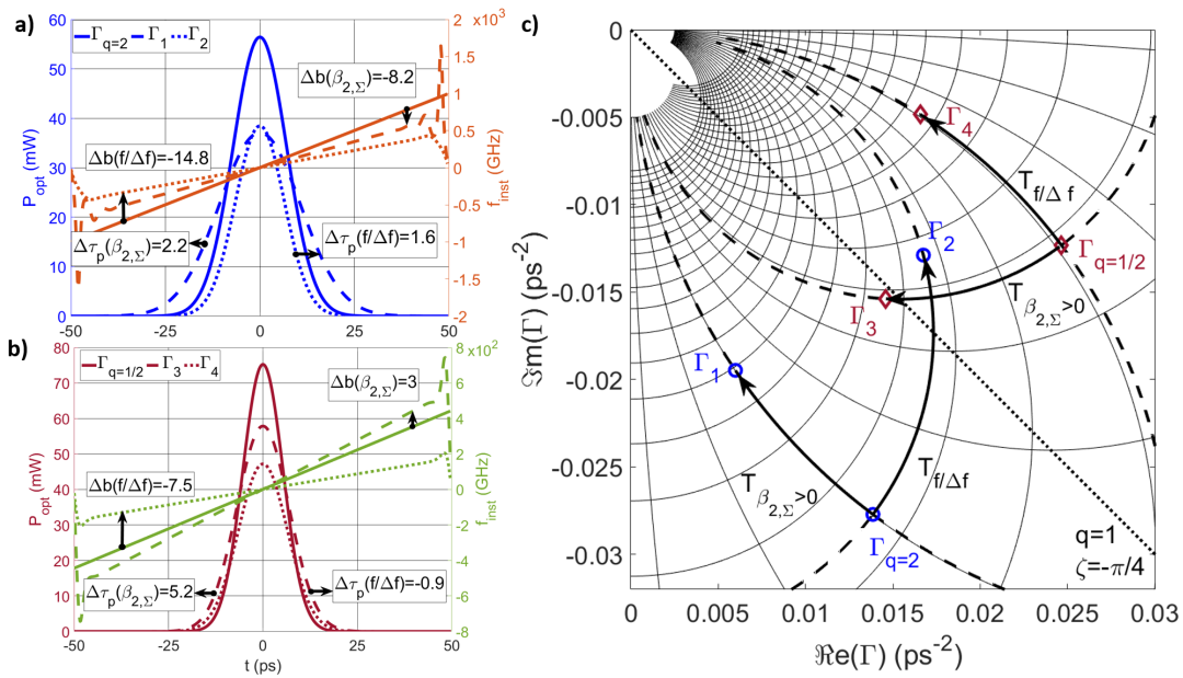
FIGURE 3.1 – Évolution d'une impulsion gaussienne \Gamma_{q=2} de paramètres \tau_p = 10 \text{ ps} , q = 2 , b = 27 \text{ GHz/ps} (a) et d'une impulsion \Gamma_{q=1/2} de paramètres \tau_p = 7.5 \text{ ps} , q = 1/2 , b = 12.3 \text{ GHz/ps} (b) sous l'effet d'une dispersion chromatique normale \beta_{2,\Sigma} = 25 \text{ ps}^2 et d'un filtre gaussien de la forme \exp(-(\omega/\Delta\omega)^2) (avec \Delta f = \Delta\omega/(2\pi) = 80 \text{ GHz} ). Les trajectoires de \Gamma sous l'effet de la dispersion chromatique ( T_{\beta_{2,\Sigma}} ) suivent des cercles de compression symétriques par rapport à l'axe des réels. Le sens de parcours des cercles est déterminé par le signe de \beta_{2,\Sigma} . Les trajectoires T_{f/\Delta f} obtenues par filtrage suivent quant à elles des cercles d'extension symétriques par rapport à l'axe des imaginaires. Les effets de filtrage et de dispersion dépendent du paramètre q de l'impulsion initiale et peuvent mener à une compression des impulsions par filtrage ainsi qu'une compensation d'un chirp positif par dispersion normale dans le cas où q > 1 . Le cas q < 1 mène à une dilatation des impulsions par filtrage et une accentuation du chirp par dispersion. Les variations de chirp et de largeur sont indiquées par \Delta b (GHz/ps) et \Delta\tau_p (ps) sur les figures a) et b) pour chacune des transformations.
