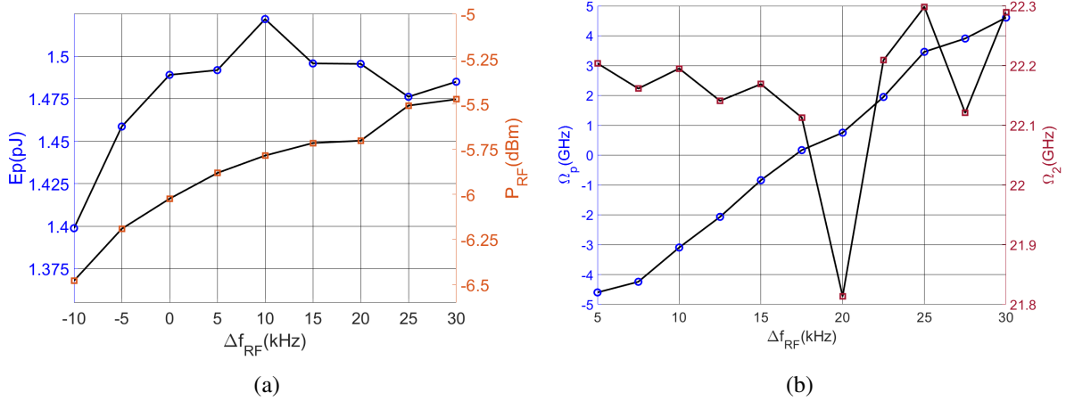
FIGURE 5.7 – a) Mesure du niveau de puissance RF et d'énergie impulsionnelle suivant le detuning. b) Évolution de la porteuse optique \Omega_p et de la largeur du spectre optique \Omega_2 mesurées.
