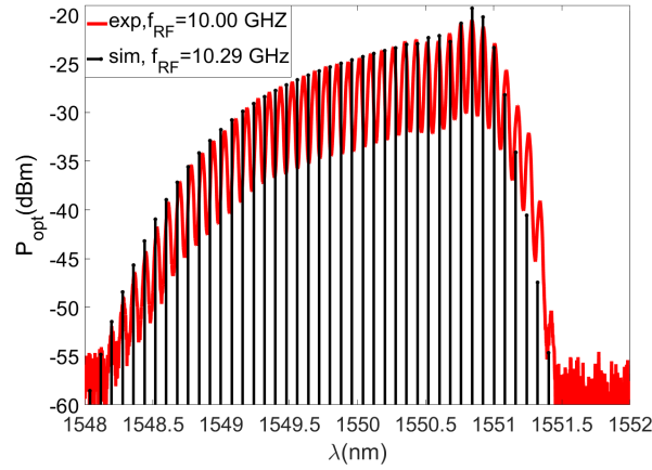
FIGURE 5.29 – Spectre optique simulé pour une dispersion \beta_{2,\Sigma} = 1.18 \text{ ps}^2 et comparé au spectre mesuré pour un COEO-AM avec waveshaper (spectre identique à celui présenté Fig.5.28) . Le waveshaper permettant une meilleure gestion de la dispersion chromatique intra-cavité que le CFBG, on retrouve des spectres optiques similaires à ceux obtenus numériquement pour la même valeur de dispersion chromatique intra-cavité. Le spectre optique expérimental a été décalé suivant \lambda et P_{opt} de sorte à ce que sa forme spectrale puisse être comparée à celle simulée. L'utilisation d'un résonateur RF centrée autour de 10.29 GHz induit un écart d'ISL du peigne expérimental par rapport au 10 GHz d'ISL simulé.
