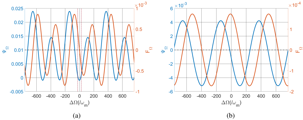
FIGURE 3.24 – a) Potentiel \Psi_\Omega calculé sur trois périodes T_\Omega dans le cas d'un COEO avec filtre optique. b) \Psi_\Omega calculé sous les mêmes conditions que a) avec un COEO sans filtre optique.
