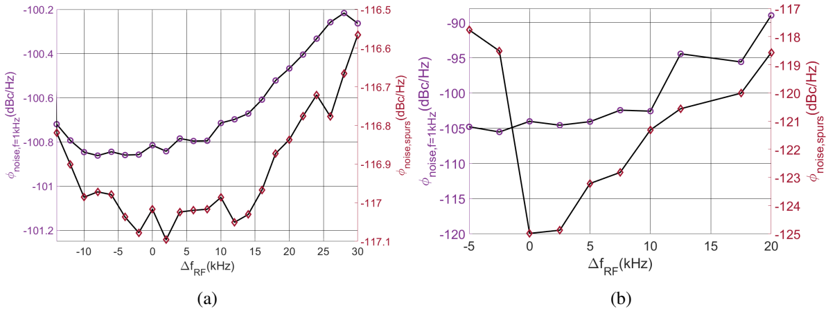
FIGURE 5.8 – Simulation (a) et mesure (b) du bruit de phase du COEO à 1 kHz de la porteuse ainsi que l'amplitude des pics des corrélations suivant \Delta f_{RF} pour une dispersion intra-cavité de \beta_{2,\Sigma,exp} = -4.32 ps^2 (avec incertitude CFBG) et \beta_{2,\Sigma,sim} = -5 ps^2 .
