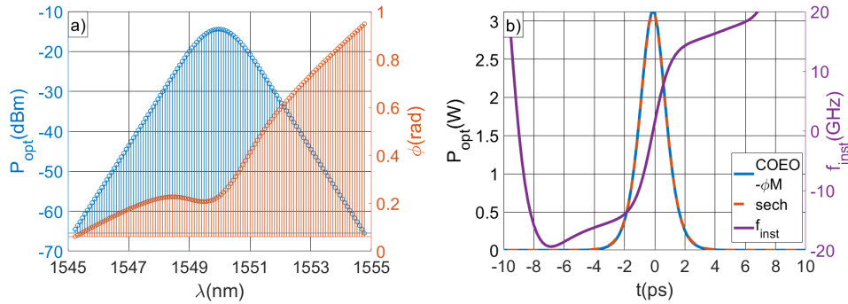
FIGURE 3.59 – a) Spectre optique du soliton obtenu par simulation du COEO- \phi M -EDFA, pour un detuning nul ( \Delta f_{RF} = 0 \text{ kHz} et une dispersion \beta_{2,\Sigma} = -0.51 \text{ ps}^2 ). b) Profil impulsionnel associé au spectre optique présenté figure a), comparé avec l'expression littérale du soliton : A(t) = A_0 \text{sech}\left(\frac{t-\xi}{\tau_p}\right) (avec \xi et \tau_p calculé à partir de l'impulsion simulée). La fréquence instantanée associée au profil impulsionnel simulé indique une impulsion à chirp positif proche de zéro (comparée aux chirps obtenus avec un COEO- \phi M -SOA, voir Fig.3.53).
