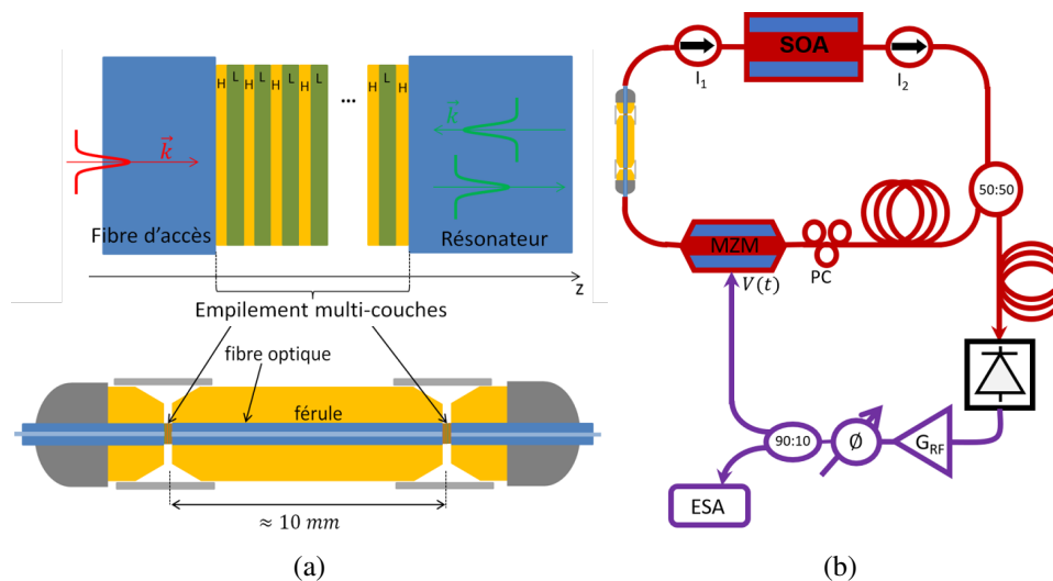
FIGURE 5.26 – a) Représentation schématique du mini-résonateur. Le dépôt de filtre de Bragg de part et d'autre du mini-résonateur permet la formation d'une cavité Fabry-Perot centrée autour des 1550 nm. Ce dernier est inséré dans le COEO (fig.b) en remplacement du filtre passe-bande optique et du résonateur RF.
