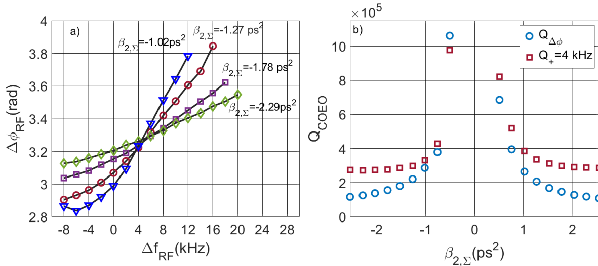
FIGURE 4.18 – a) \Delta\phi(\Delta f_{RF}) simulé et mesuré pour différentes valeurs de dispersion chromatique anormale intra-cavité. La pente de phase permet de calculer le facteur de qualité mesurable expérimentalement Q_{\Delta\phi} . b) Évolution du facteur de qualité Q_{\Delta\phi} suivant \beta_{2,\Sigma} , comparé au facteur de qualité Q_+ pour un detuning de 4 kHz. Q_{\Delta\phi} suit l'évolution qualitative de Q_+ .
