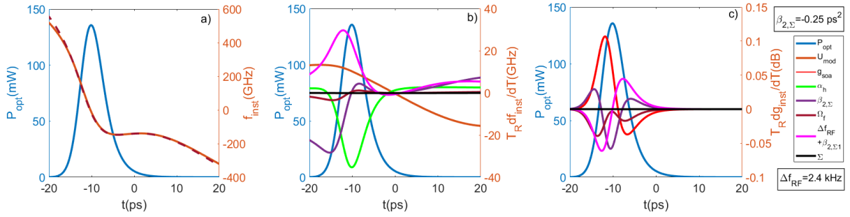
FIGURE 3.53 – a) Profil d'intensité optique ainsi que la fréquence instantanée associée. La courbe f_{inst} en pointillées correspond à la fréquence instantanée reconstituée à partir de la méthode des moments. La courbe f_{inst} pleine a été obtenue à partir de la définition : f_{inst} = -\frac{1}{2\pi} \frac{d\phi}{dt} . b) Contribution par tour de cavité des composants de la boucle optique au profil de fréquence instantanée. c) Contribution des composants optiques au gain instantané perçu par l'impulsion. Les courbes \Sigma donnent la somme des contributions individuelles de chacun des composants.
