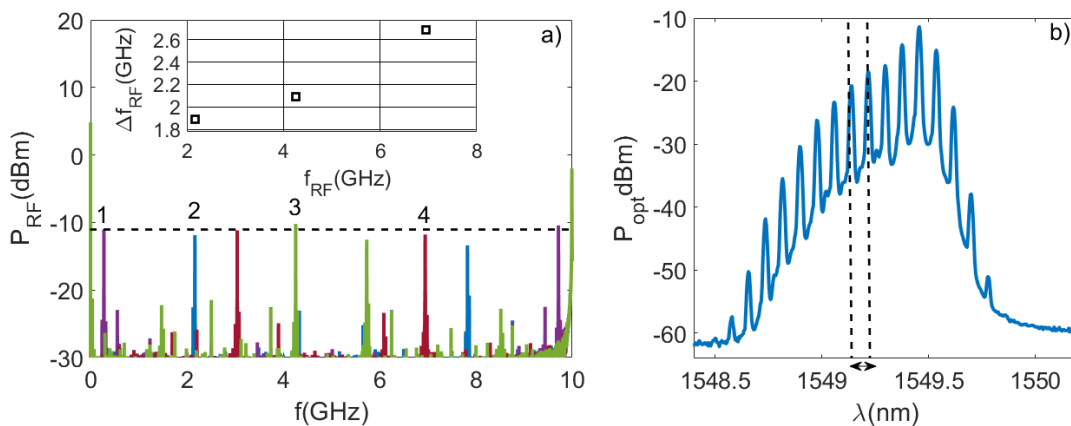
FIGURE 5.20 – a) Évolution du spectre de battement obtenue par transformée de Fourier de l'acquisition de l'oscilloscope à temps réel lors du parcours d'un ISL du peigne optique par le laser accordable. Les battements numérotés de 1 à 4 (violet, bleu, vert et rouge) sont issus des quatre acquisitions de spectres réalisées pour chaque ISL. La ligne horizontale indique le niveau du premier battement afin d'estimer les variations de puissance RF lors du parcours de l'ISL. b) Peigne de fréquence du COEO participant aux battements présentés Fig.a). Le Laser accordable balaye l'ISL délimité en pointillé. \Delta f_{RF} donne l'évolution du pas effectué par la fréquence de battement à chaque nouvelle position du laser. Le spectre optique présenté a été obtenu pour une dispersion intra-cavité D = 14\text{ ps/nm} .
