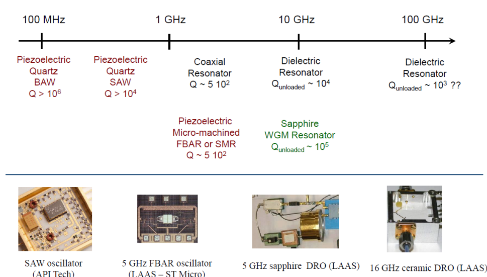
FIGURE 1.1 – Évolution des facteurs de qualité des résonateurs RF et de leur technologie suivant la fréquence de résonance.
