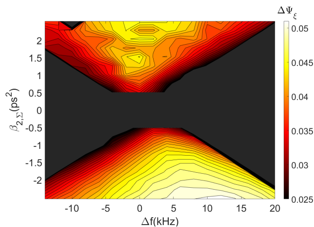
FIGURE 3.35 – Dépendance de la barrière de potentiel \Delta\Psi_\xi suivant le detuning \Delta f et la dispersion chromatique \beta_{2,\Sigma} . La bande de verrouillage s’élargit en forme de V de manière analogue aux langues de Arnold pour un rapport 1/1 obtenu avec l’équation d’Adler (Fig.3.34). La dispersion chromatique affecte donc le couplage entre les deux oscillateurs (noté \epsilon sur Fig.3.34), de sorte à ce que \epsilon augmente lorsque \beta_{2,\Sigma} diminue.
