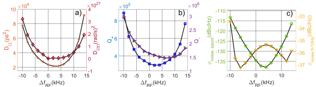
FIGURE 4.9 – Évolution suivant \Delta f_{RF} : a) des coefficients de diffusion D_{\xi\xi} , D_{\Omega\Omega} , b) des facteurs de qualité Q_{\pm} , c) de l'amplitude des pics de corrélation du bruit de phase et du bruit de phase proche porteuse ( f = 10 Hz) pour une dispersion intra-cavité \beta_{2,\Sigma} = 1.27 ps 2
