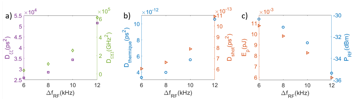
FIGURE 4.6 – Évolution des coefficients de diffusion des sources de bruit optiques (a) et RF (b). L
