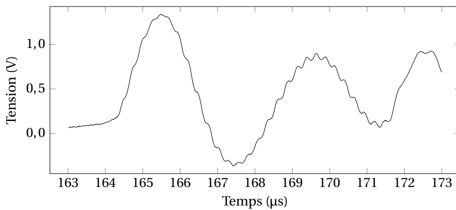
(a) Signal mesuré pour l'essai à v_{\text{impact}} = 600 \text{ m} \cdot \text{s}^{-1}
