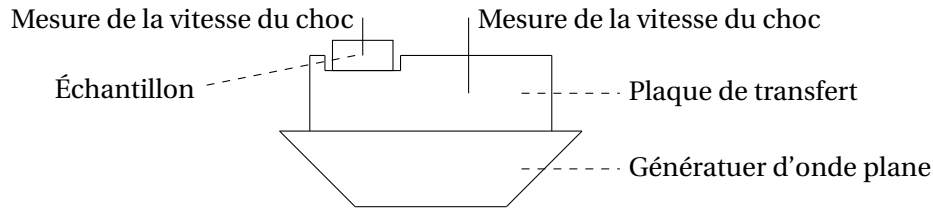
FIGURE 1.4 – Montage expérimental de DICK [10]
