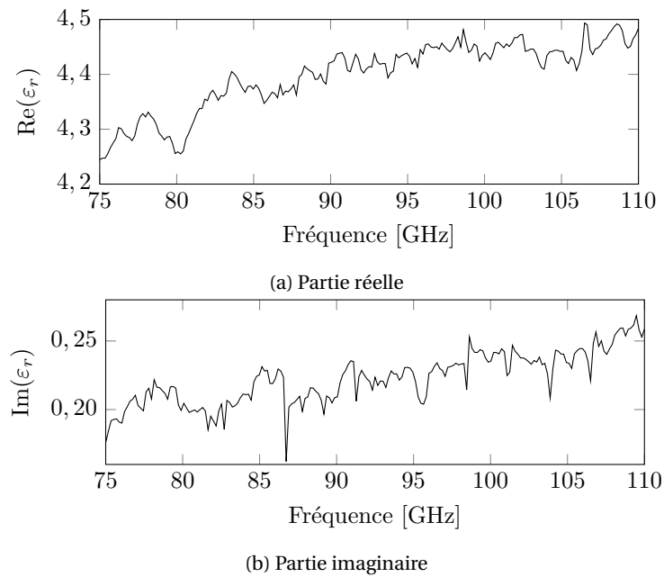
FIGURE C.3 – Permittivité complexe du mélange RDX-ONTA-Aluminium-Liant inerte
