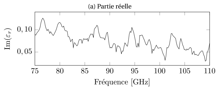
FIGURE C.1 – Permittivité complexe du mélange HMX-ONTA-Liant inerte
