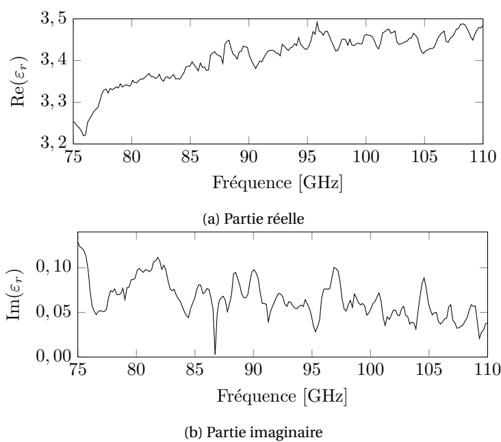
FIGURE C.14 – Permittivité complexe du mélange 2 de HMX-Liant inerte
