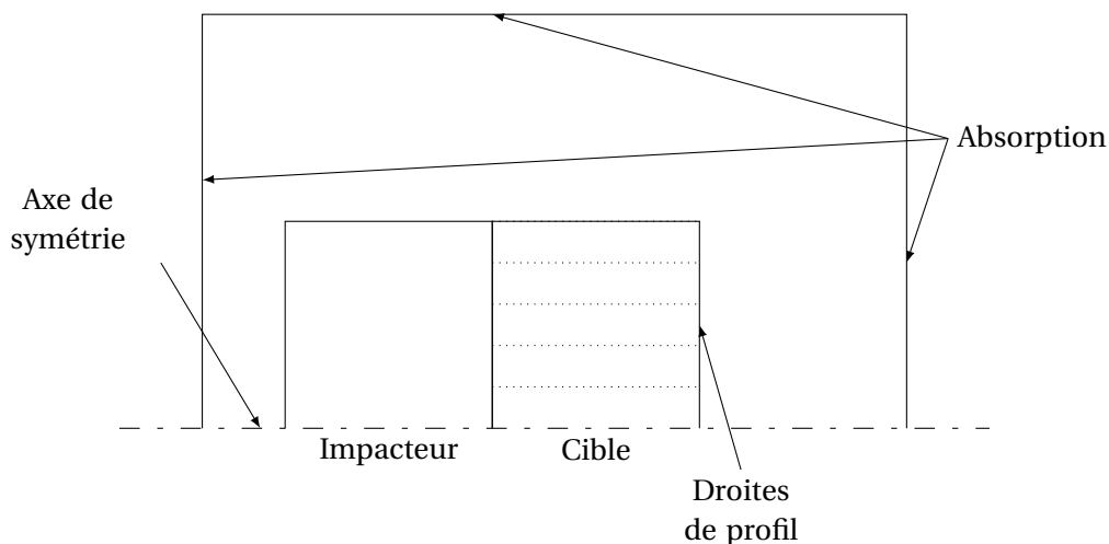
FIGURE 2.23 – Configuration de la simulation pour l'étude des détonces latérales
