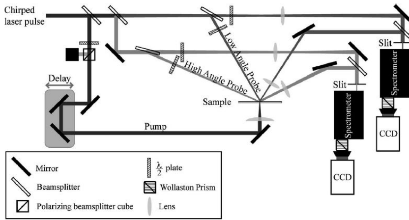
FIGURE 1.15 – Montage expérimental d'ellipsométrie dynamique [37]
