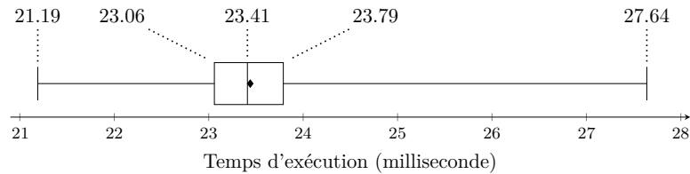
FIGURE 5.1 – Temps d'exécution de l'étape 1 (S1 et S3)
